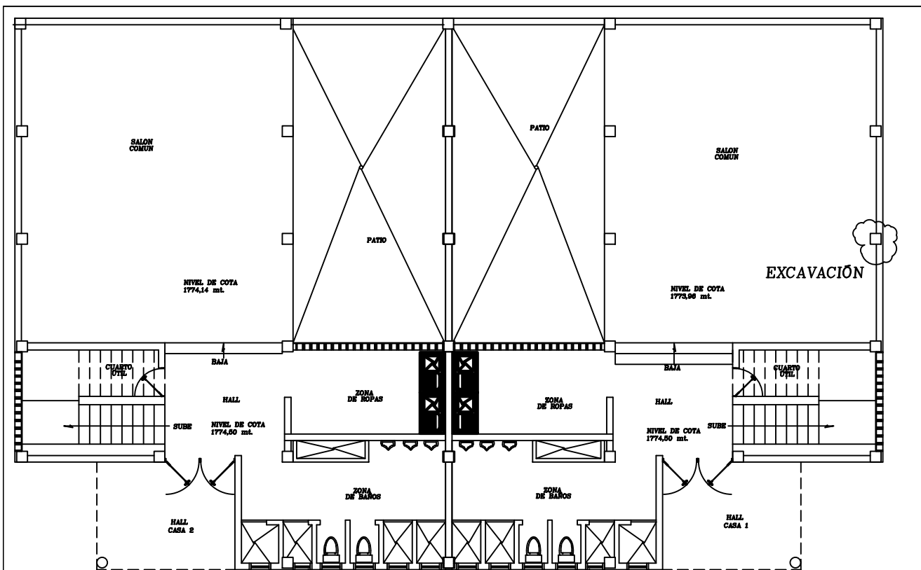
CASA 1 DETALLE DE FUNDACIÓN PLANTA PRIMER PISO CASA 1 SEDE SANTA RITA
