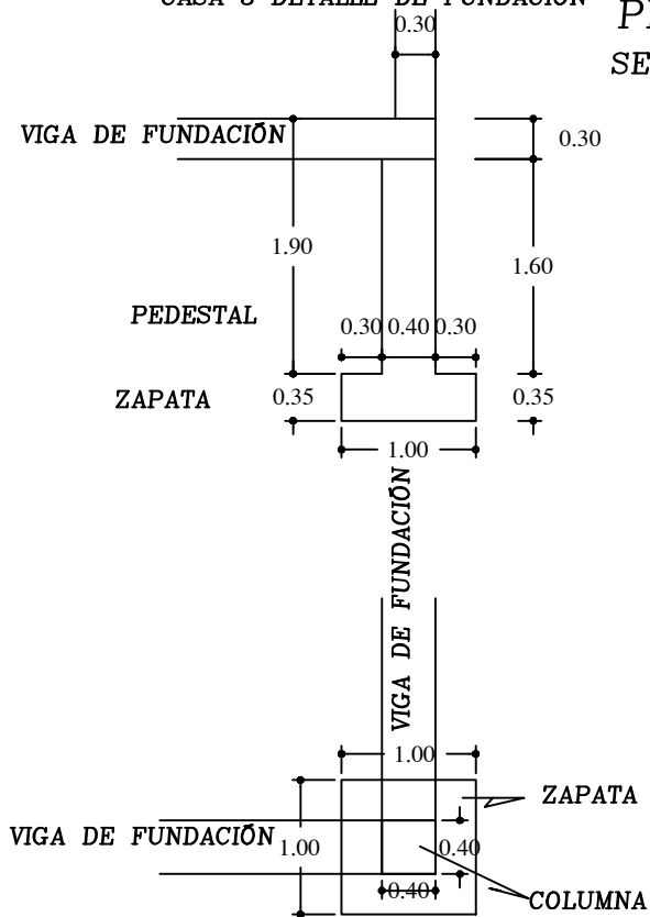
CASA 3 DETALLE DE FUNDACIÓN
