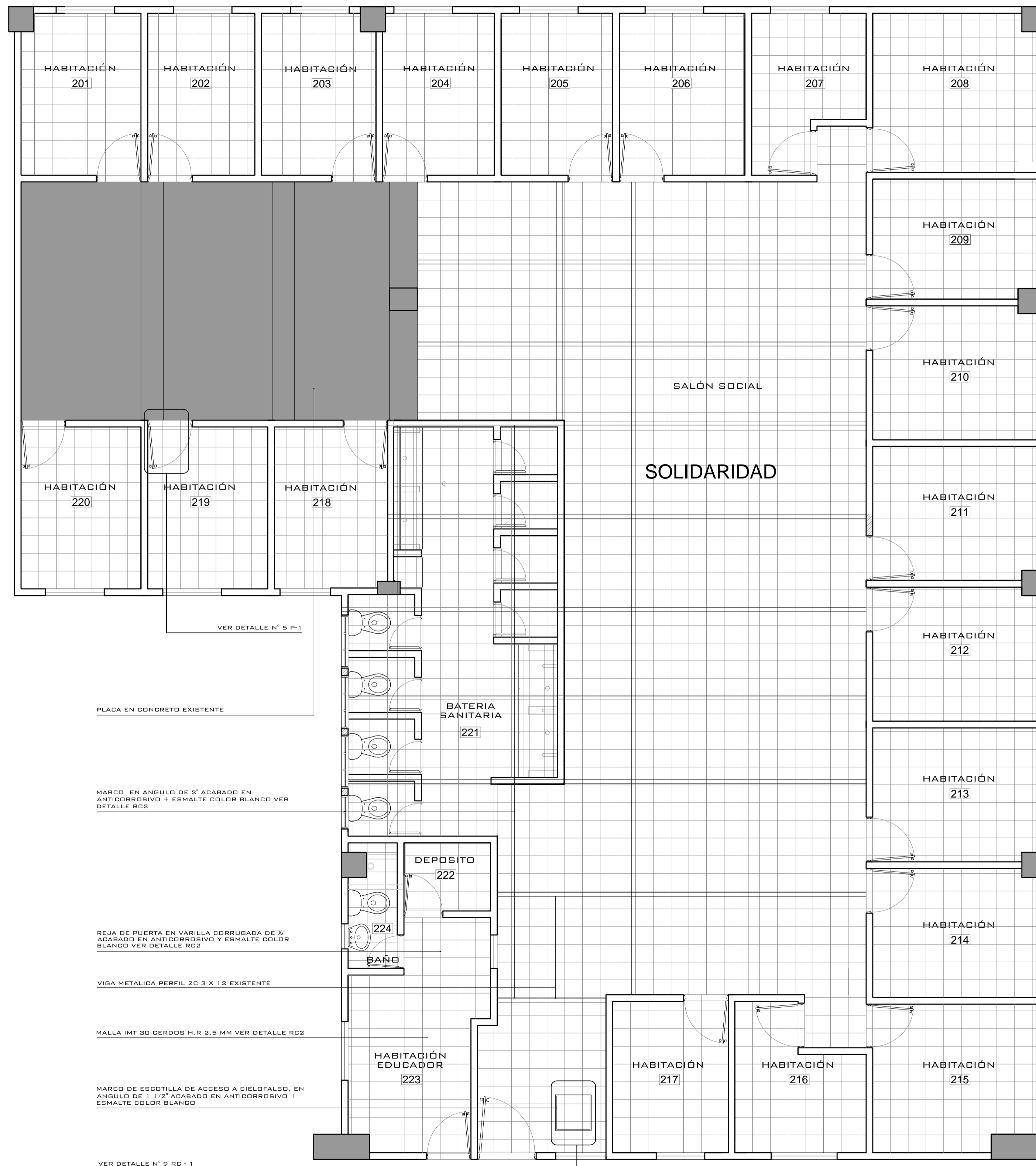
PLANTA CIELORASOS CASA SOLIDARIDAD ESC: 1:50
