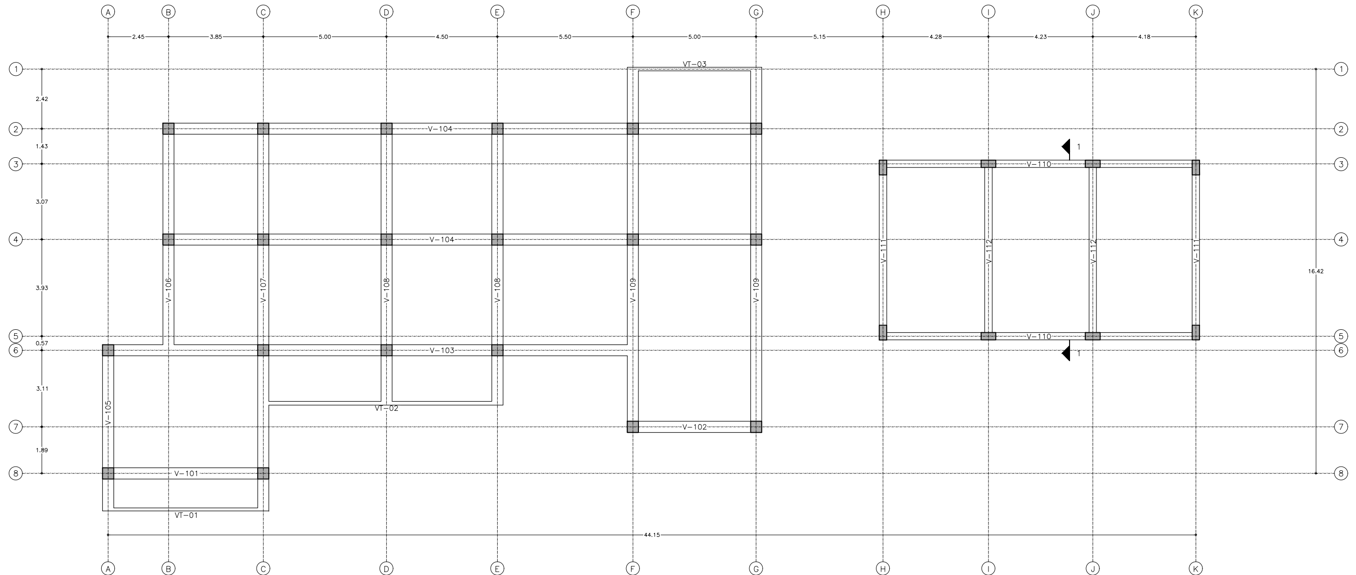
PLANTA CIMENTACIÓN NE + 0.20 Escala 1:150
