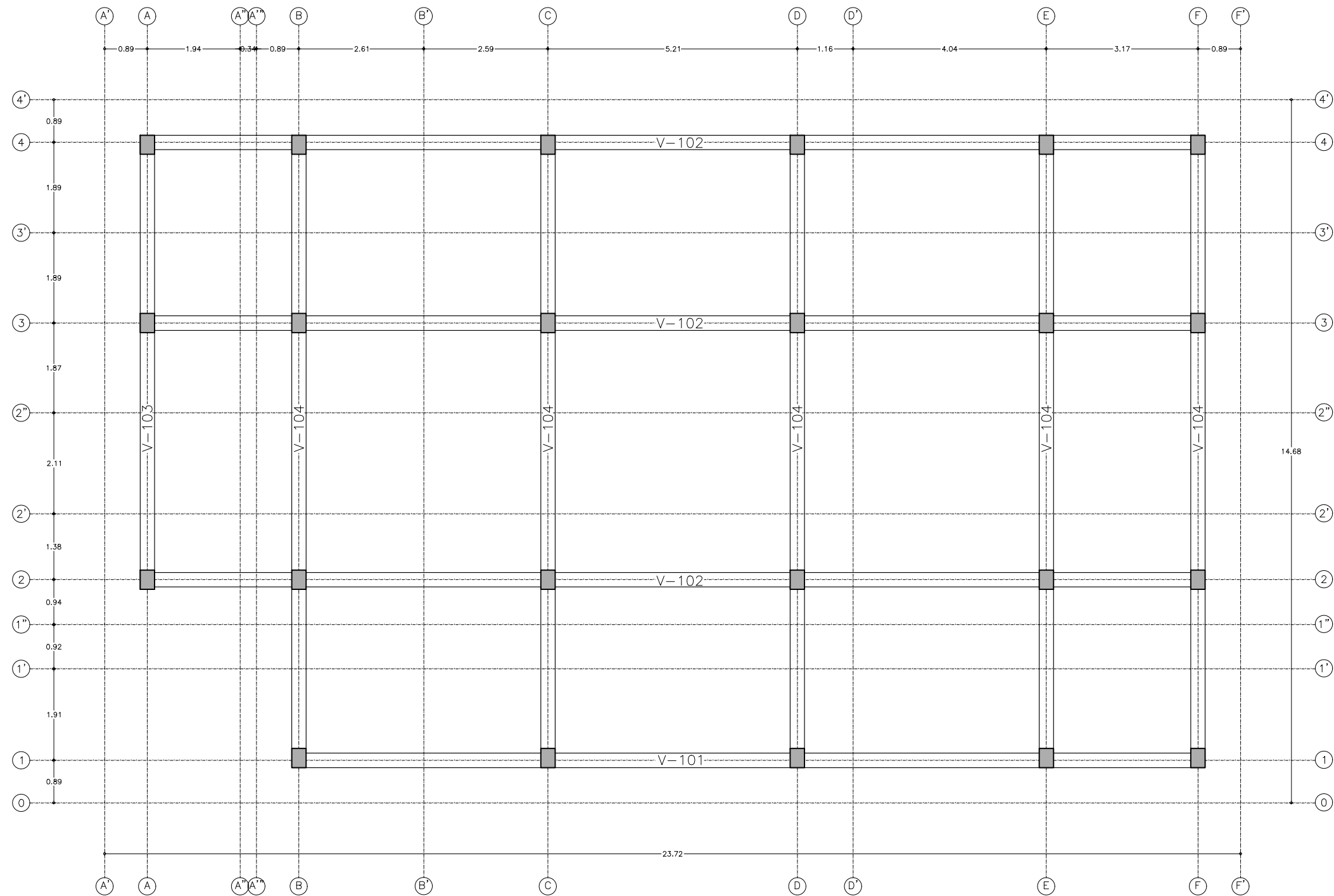
PLANTA NE +0.20 Escala 1:100
