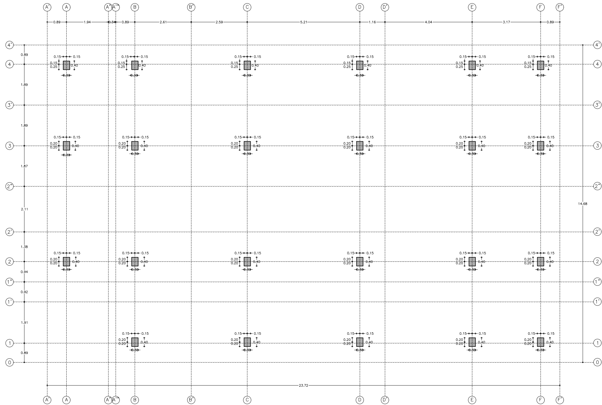
PLANTA LOCALIZACIÓN DE EJES Y COLUMNAS Escala 1:100
