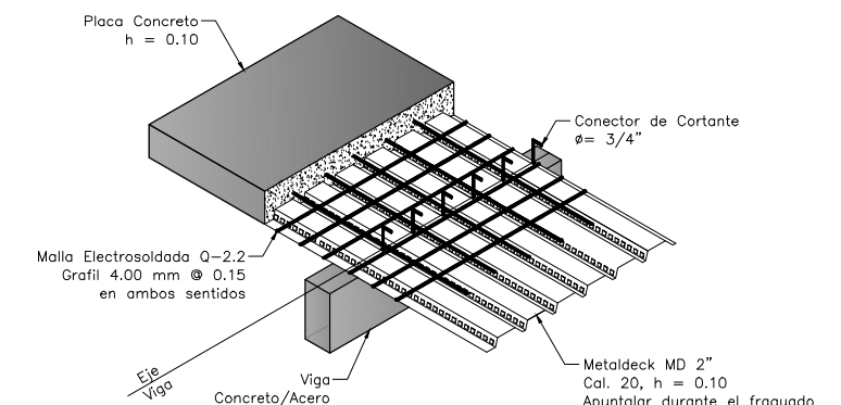
DETALLE PLACA ENTREPISO Escala 1:25
