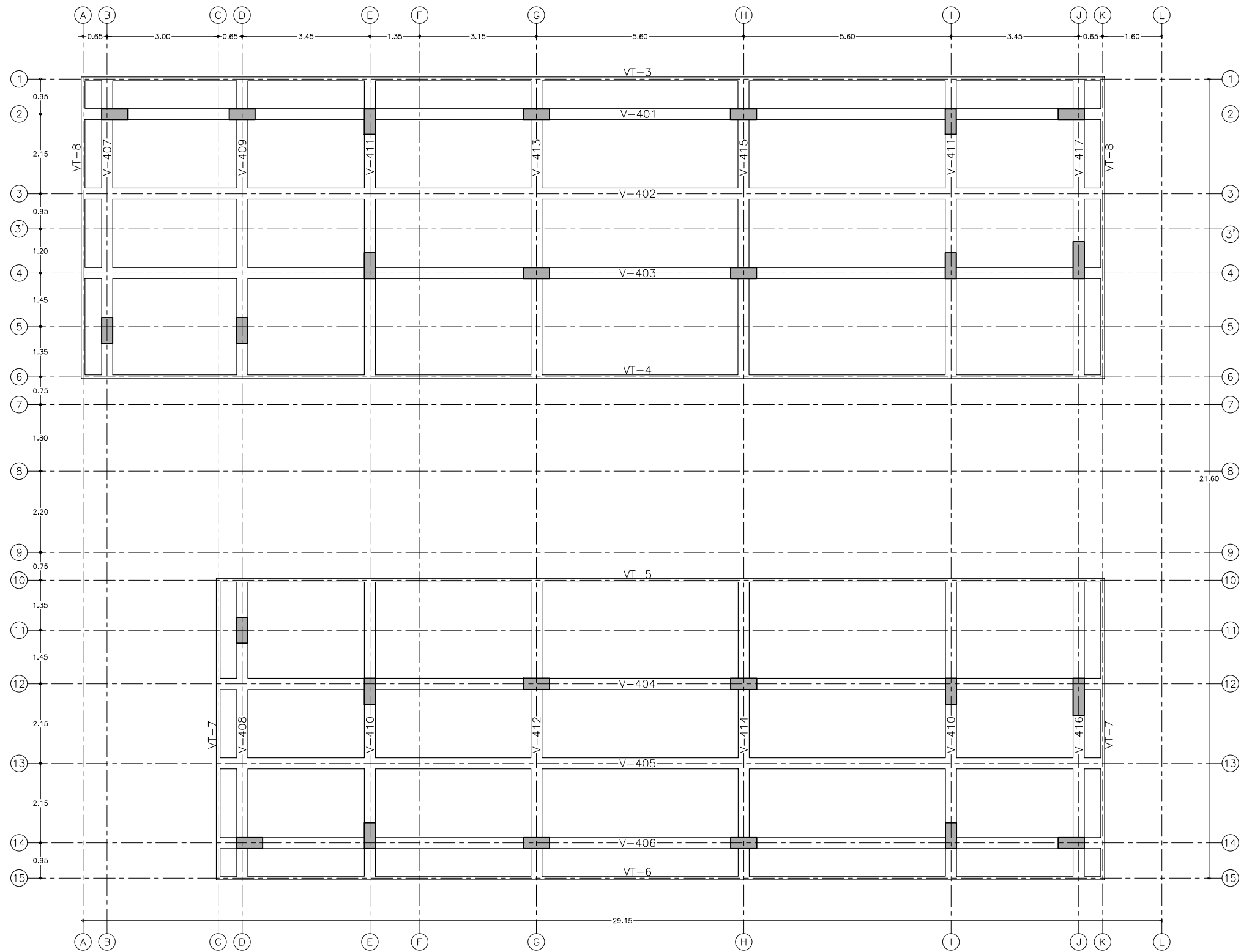
PLANTA DE CUBIERTA Escala 1:125
