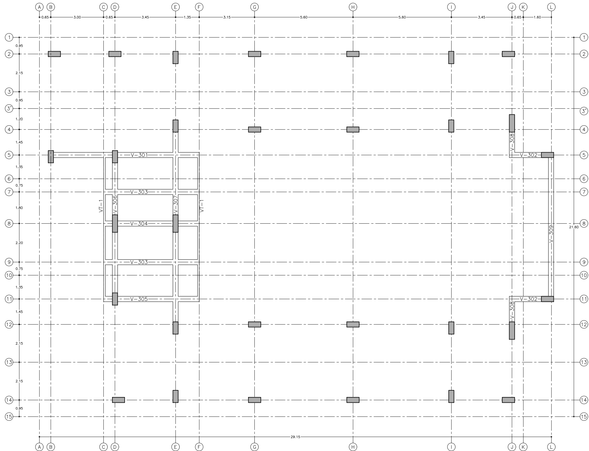
PLANTA ESTRUCTURAL, NE +9.80 Escala 1:125
