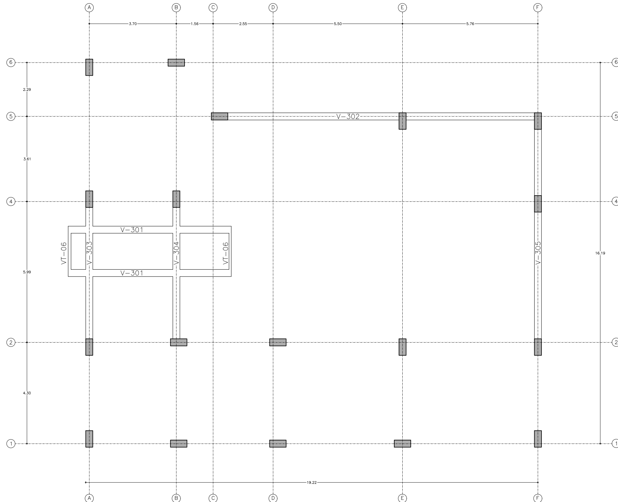
PLANTA NE +9.70
