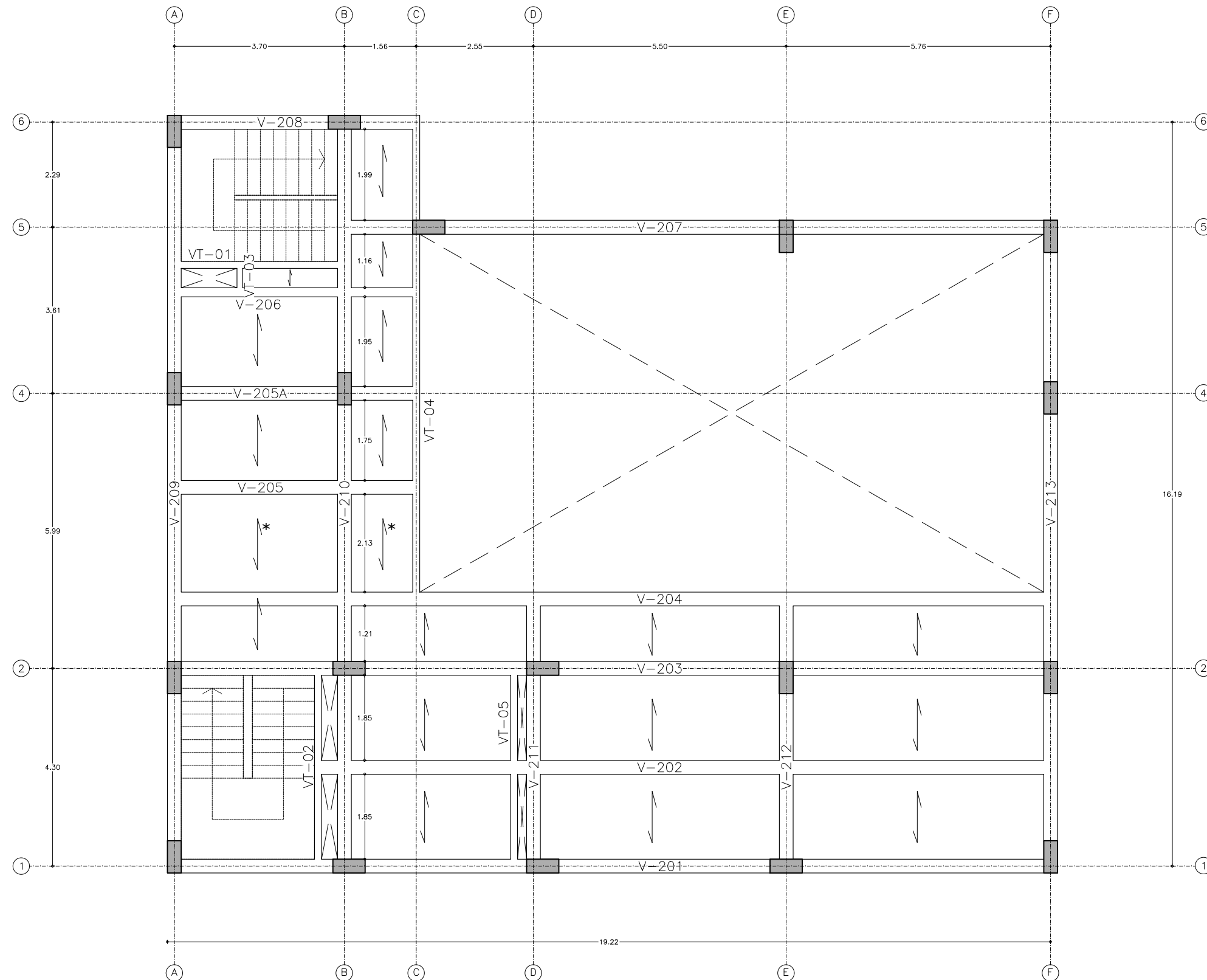
PLANTA NE +6.20 Escala 1:100
