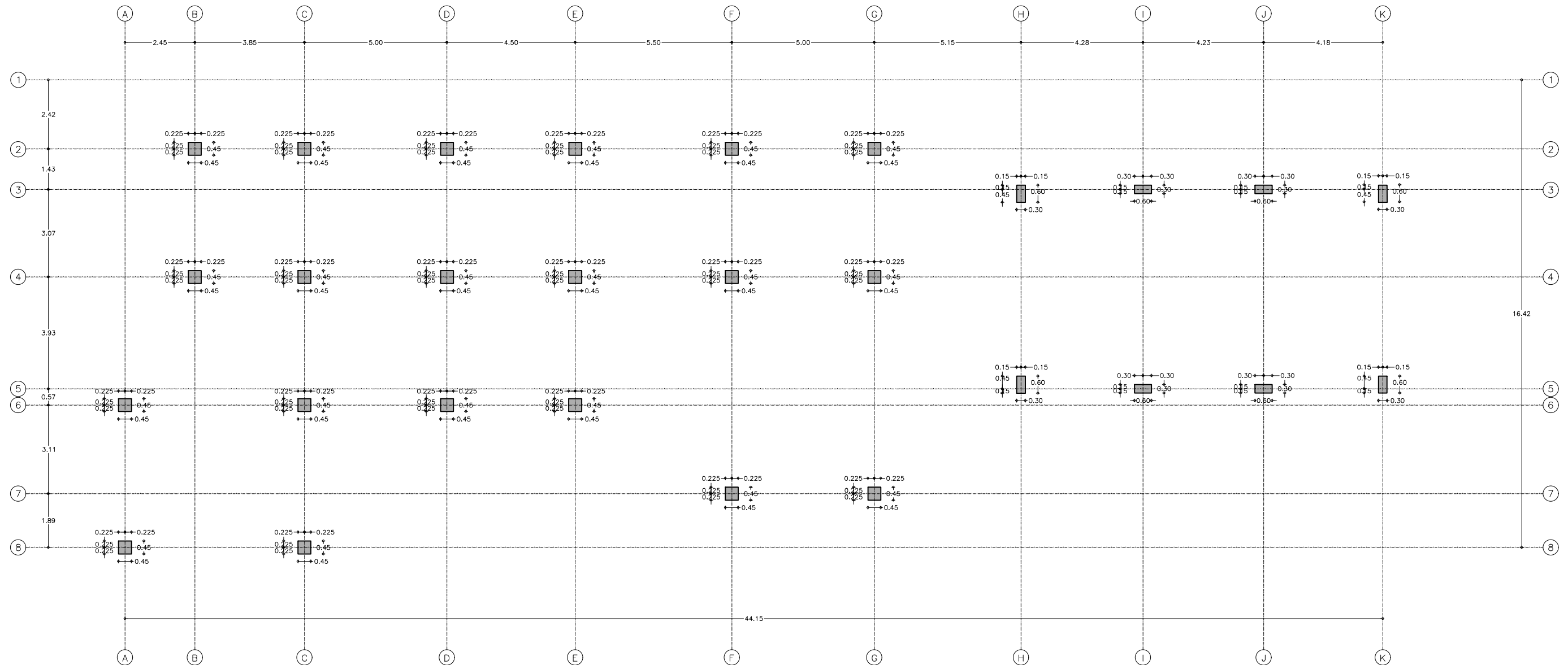
PLANTA LOCALIZACIÓN EJES Y COLUMNAS Escala 1:150
