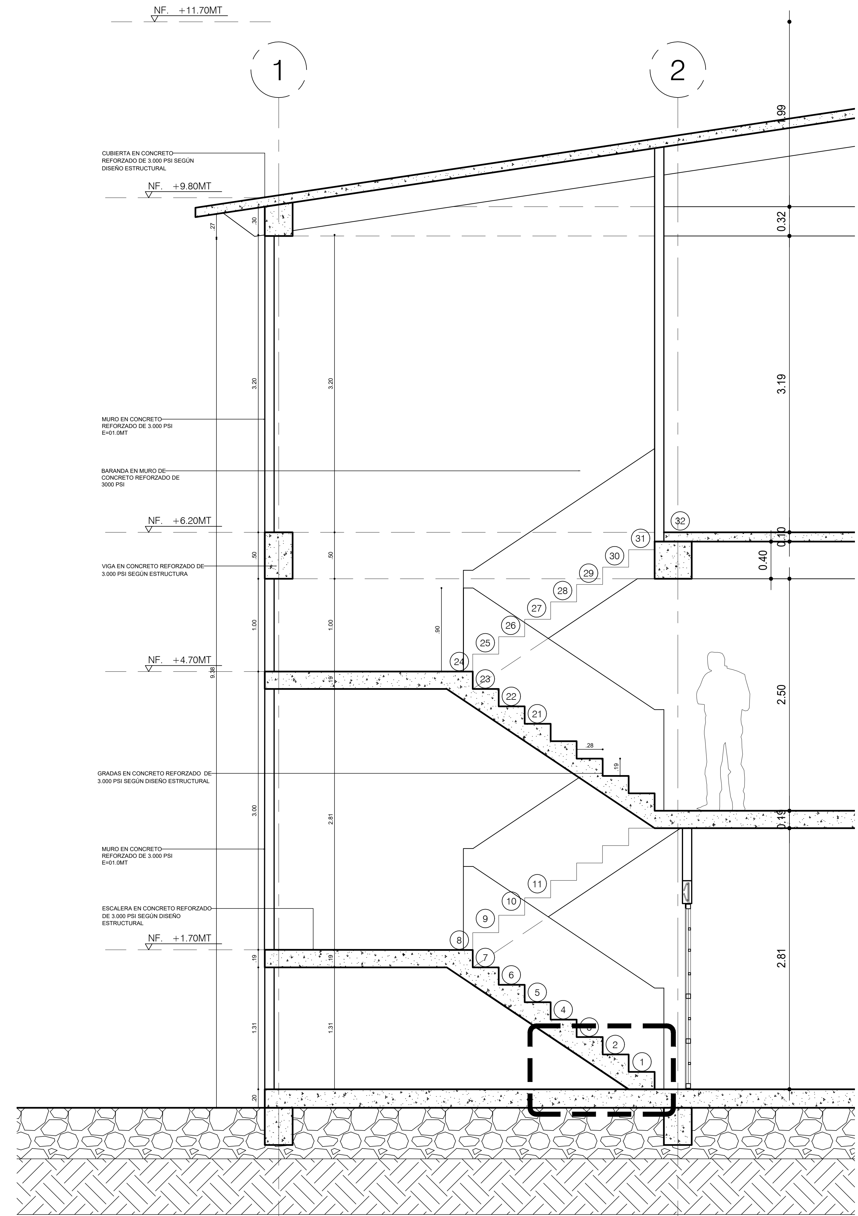
A3 DETALLE SECCION ECALERAS ESCALA 1:25
