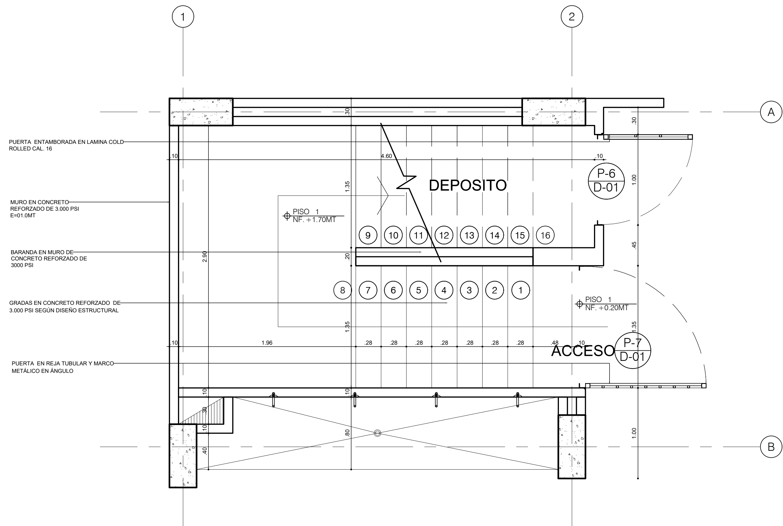
A1 DETALLE ESCALERA PLANTA ESCALA 1:25
