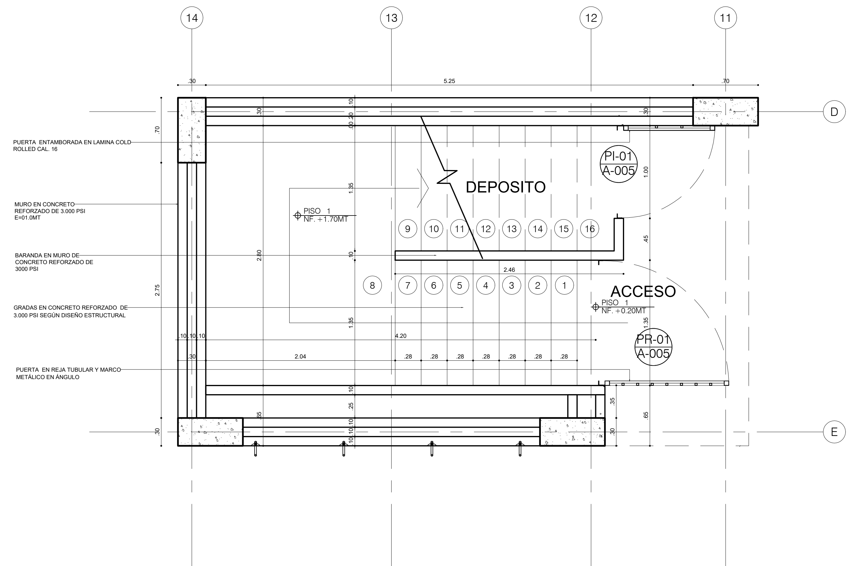
A1 DETALLE ESCALERA PLANTA ESCALA 1:25
