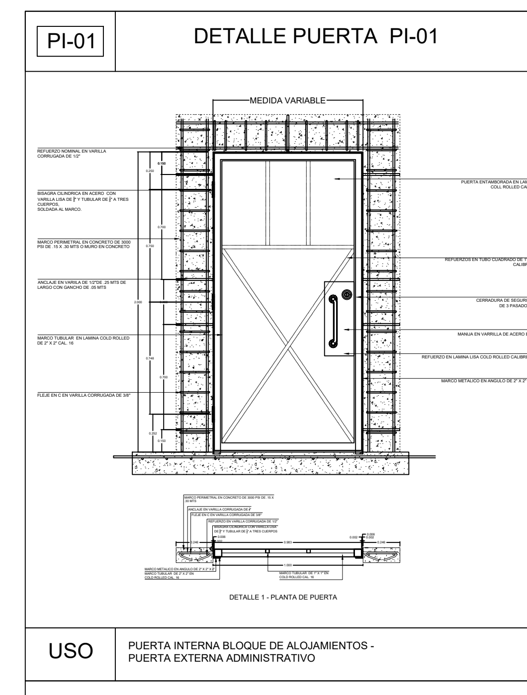
A3 DETALLE PUERTAS Y VENTANAS ESCALA 1:25
