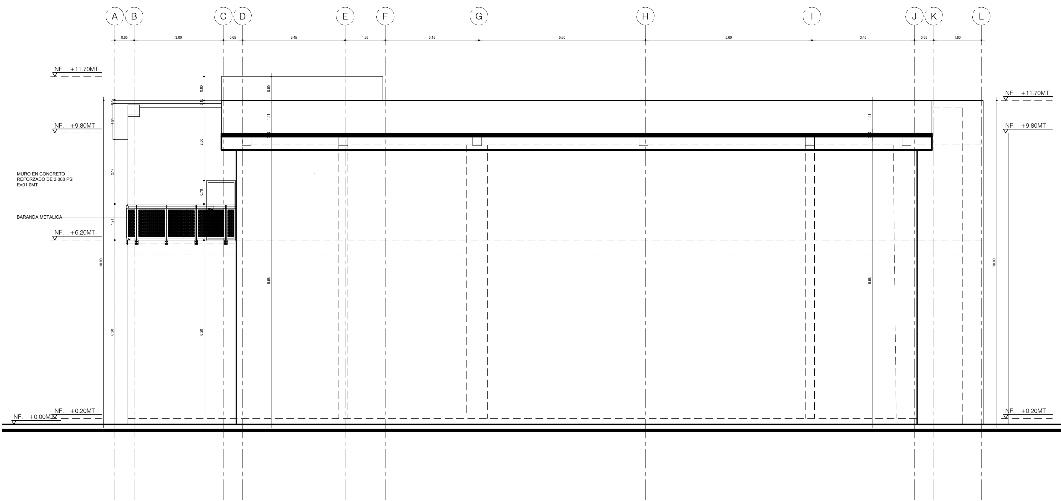
A2 FACHADA LATERAL DERECHA F3 ESCALA 1:75
