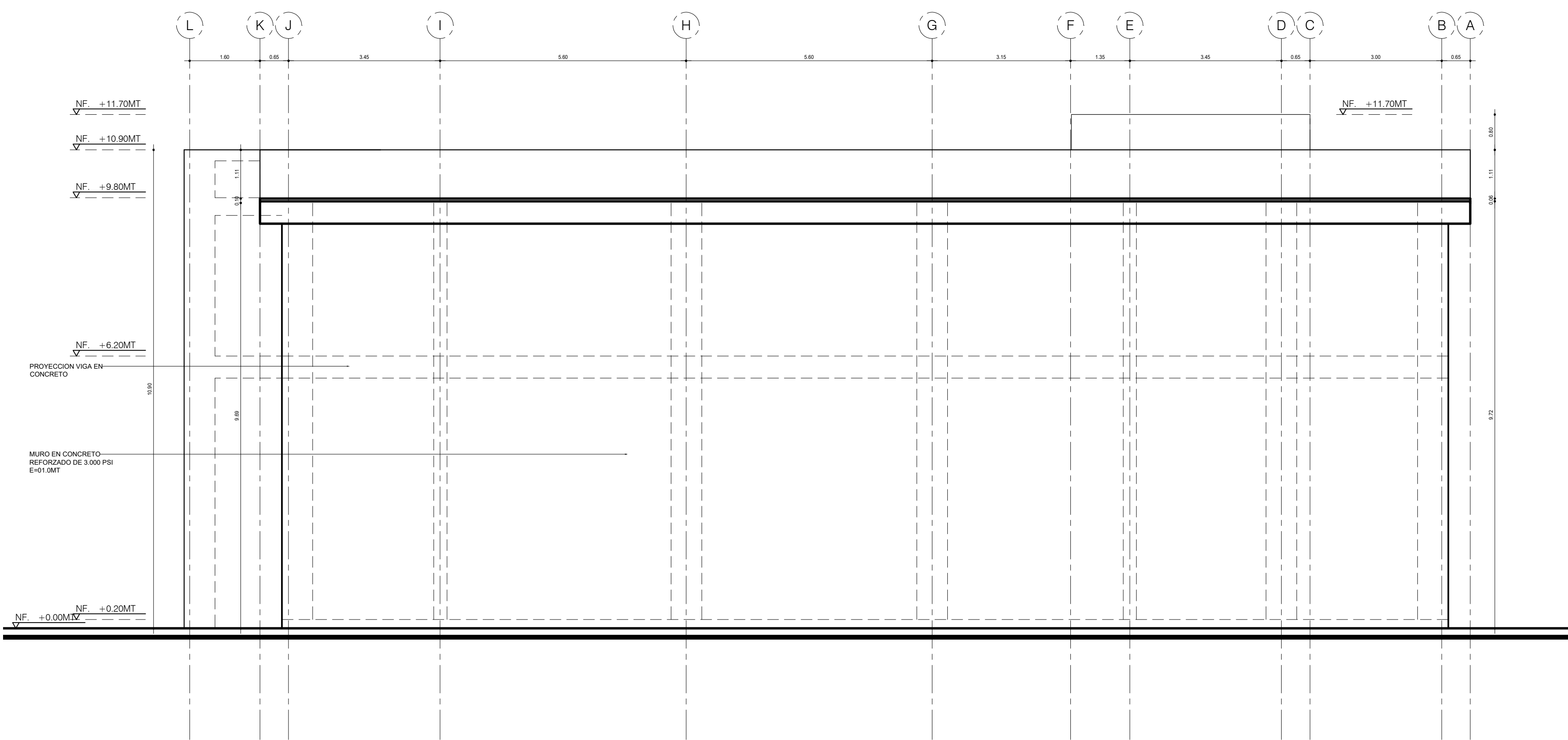
A1 FACHADA LATERAL IZQUIERDA F4 ESCALA 1:75
