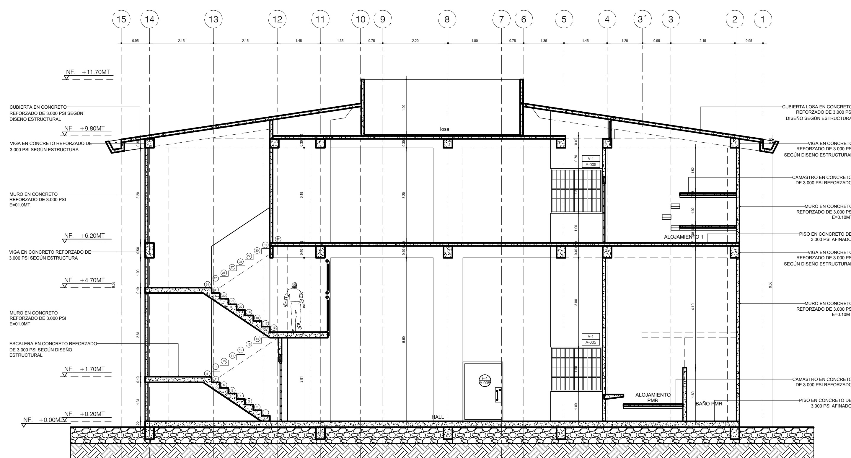
A3 CORTE B-B ESCALA 1:75
