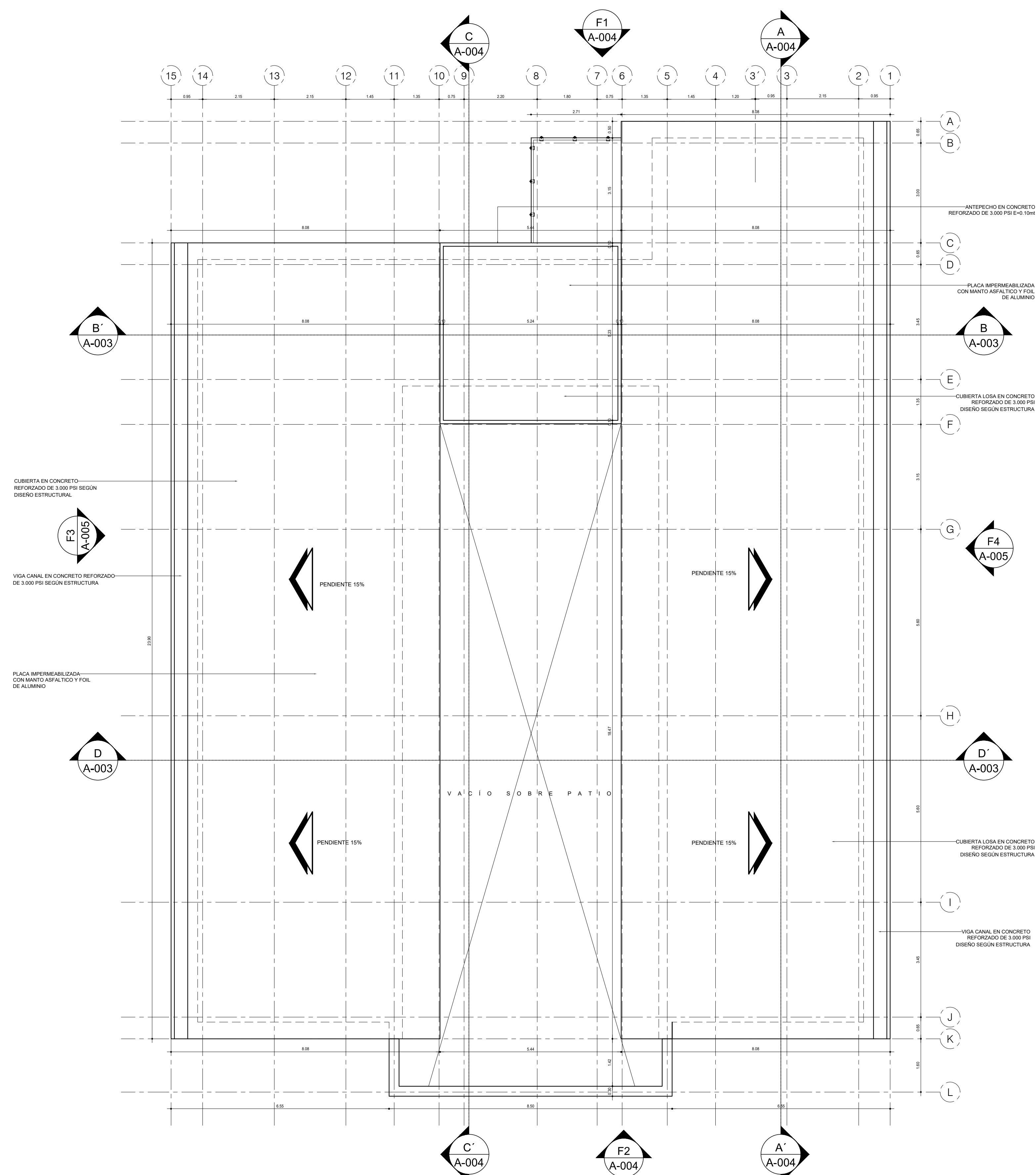
A1 PLANTA CUBIERTA ESCALA 1:75
