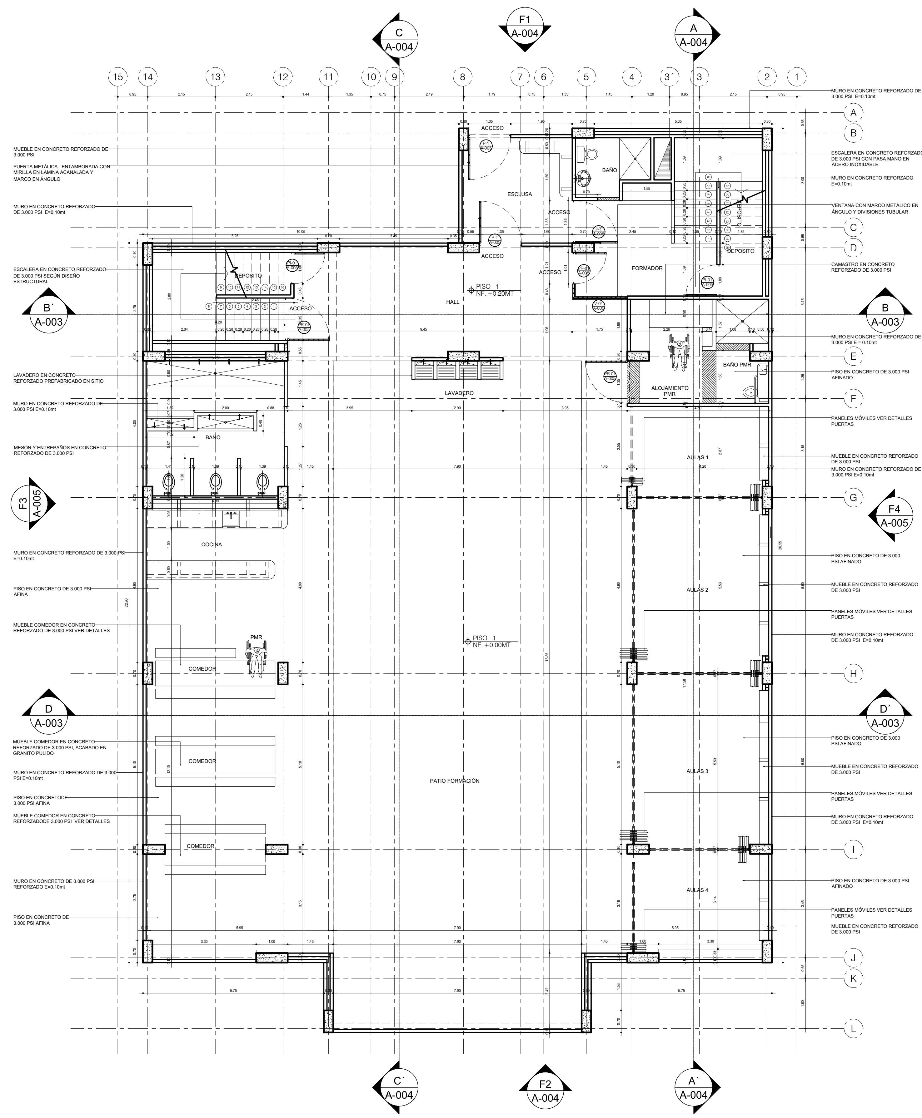
A1 PLANTA PRIMER PISO ESCALA 1:75
