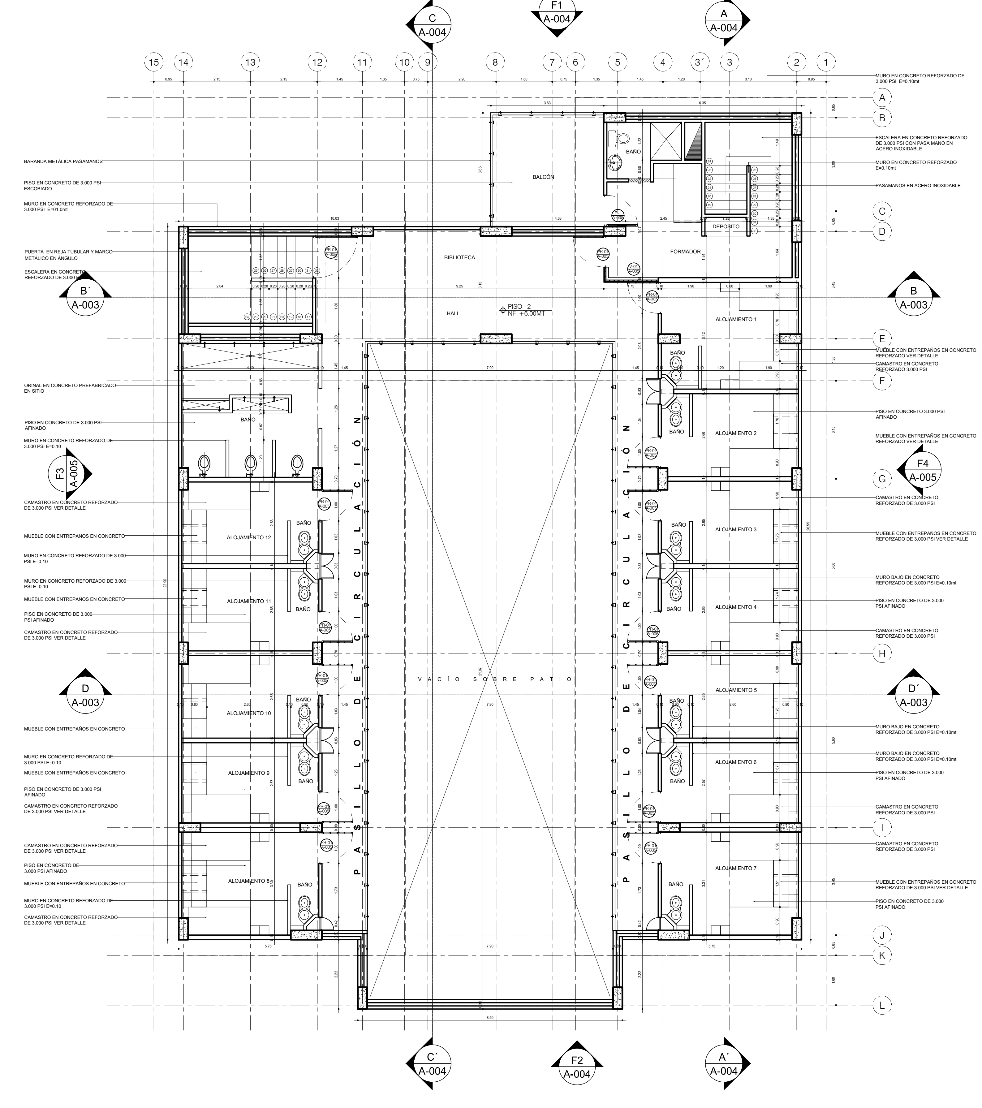
A2 PLANTA SEGUNDO PISO ESCALA 1:75
