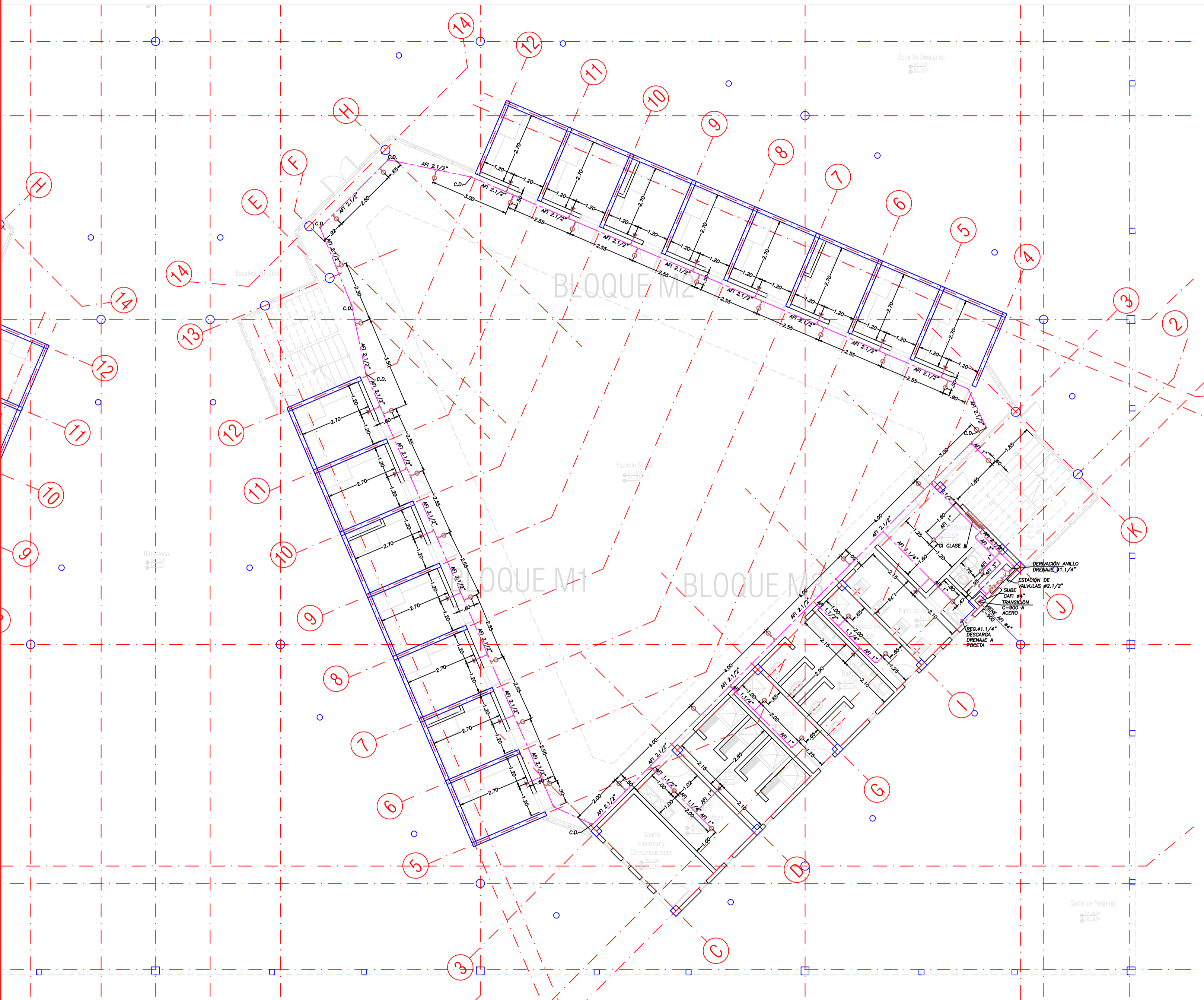
PLANTA PRIMER PISO (BLOQUE H Y M) Incendio Escala 1:75
