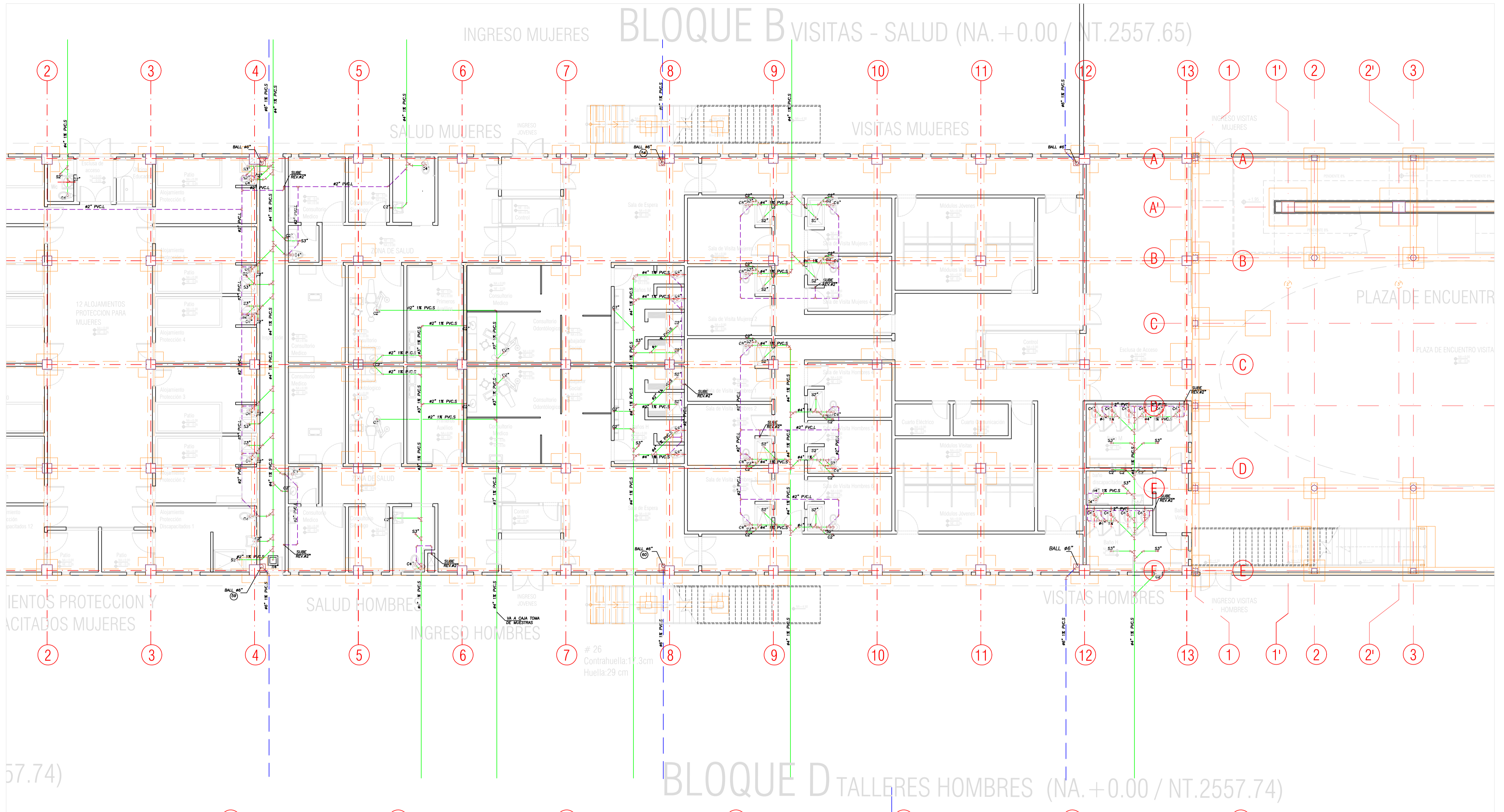
PLANTA BLOQUE CENTRAL PRIMER PISO BLOQUE B Desagues Escala 1:75
