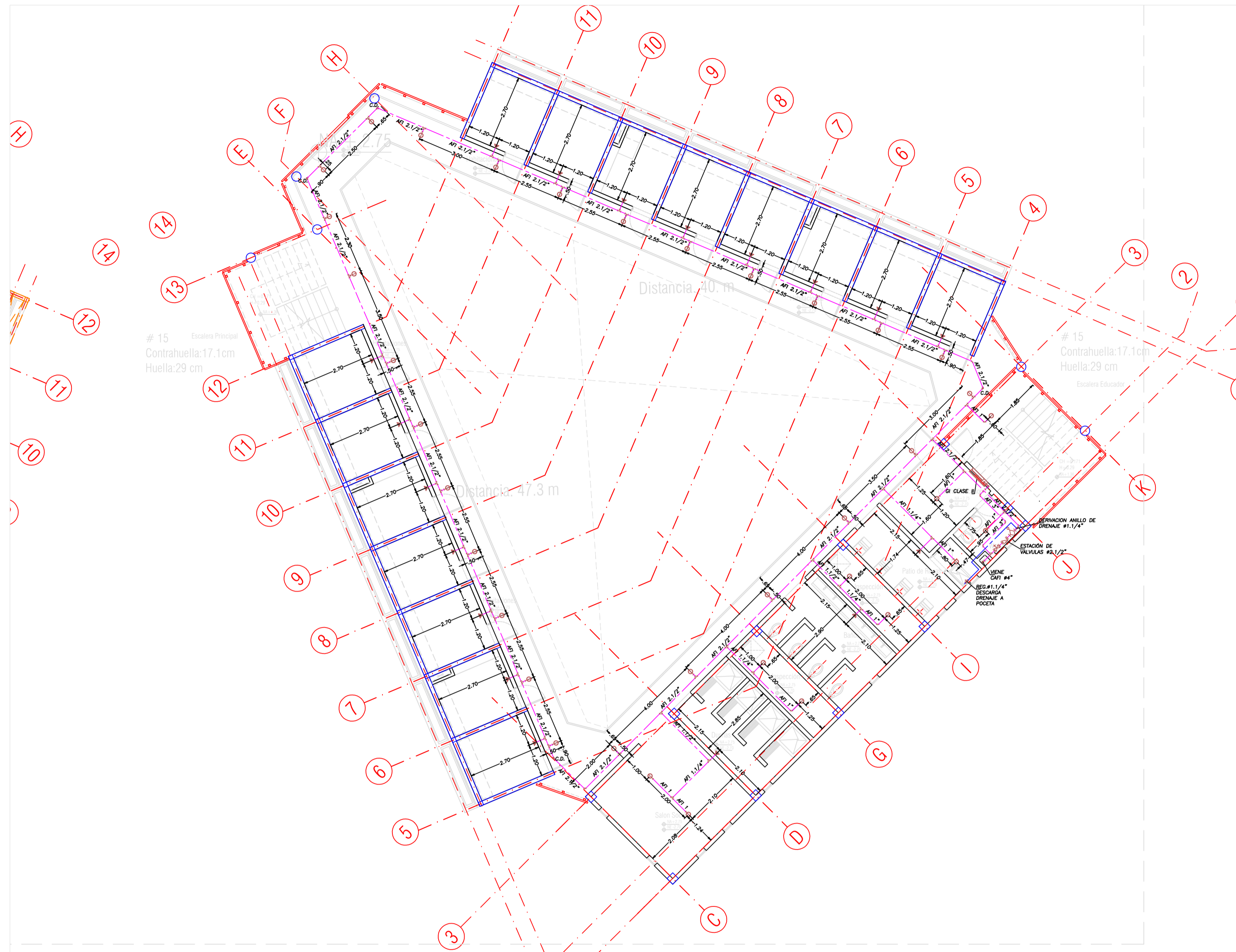
PLANTA PISO TIPO (BLOQUE H Y M) Incendio Escala 1:75
