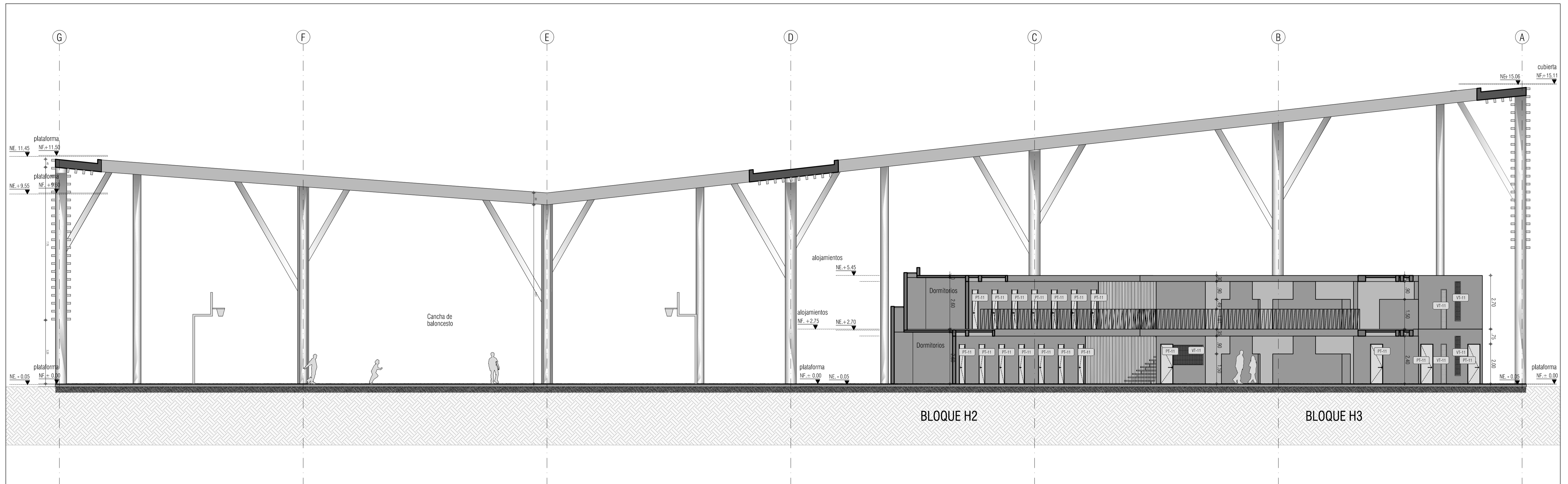
Esc 1/100 CORTE LONGITUDINAL S-S' / ALOJAMIENTO MUJERES
