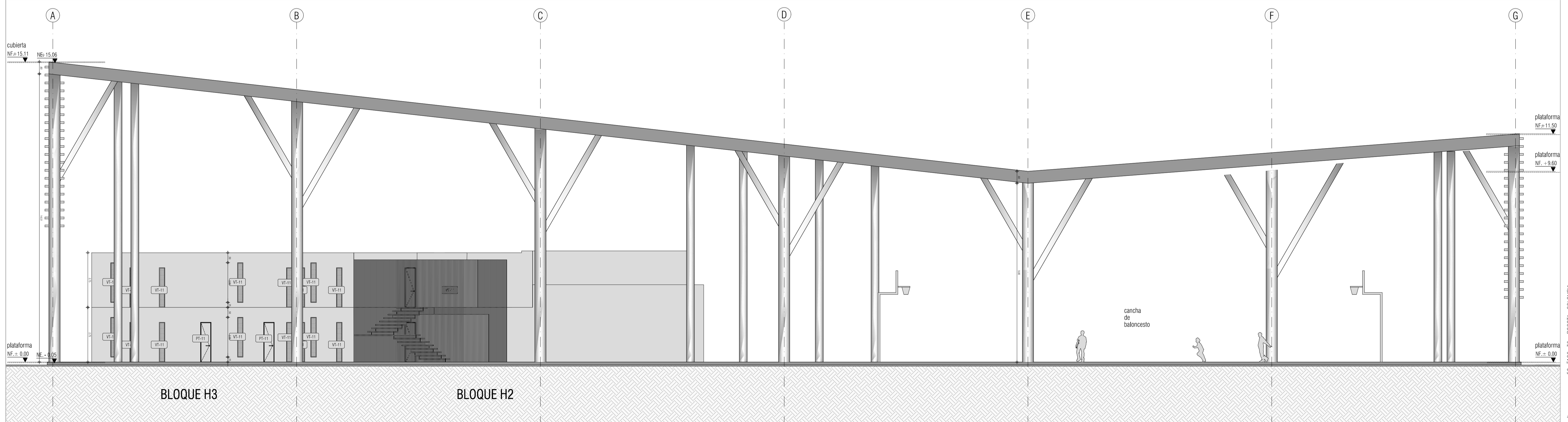
Esc 1/100 FACHADA SUR / ALOJAMIENTO MUJERES
