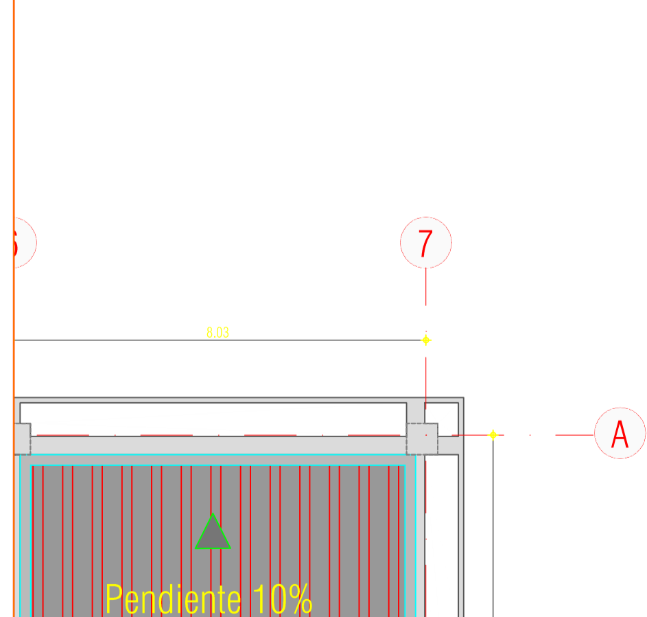
PLANTA CUBIERTA BLOQUE A ESC. 1:100
