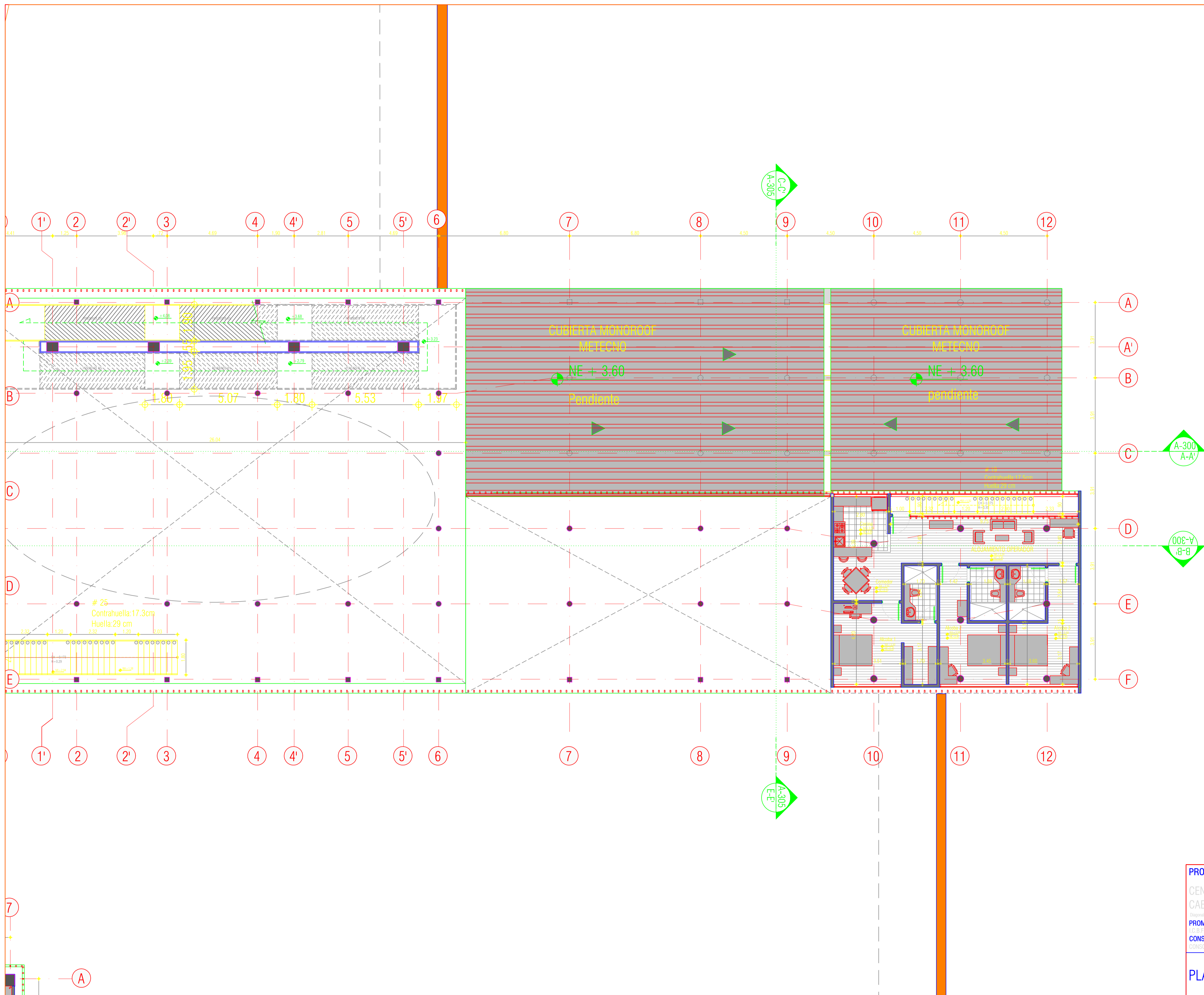
PLANTA SEGUNDO PISO BLOQUE A ESC. 1:100
