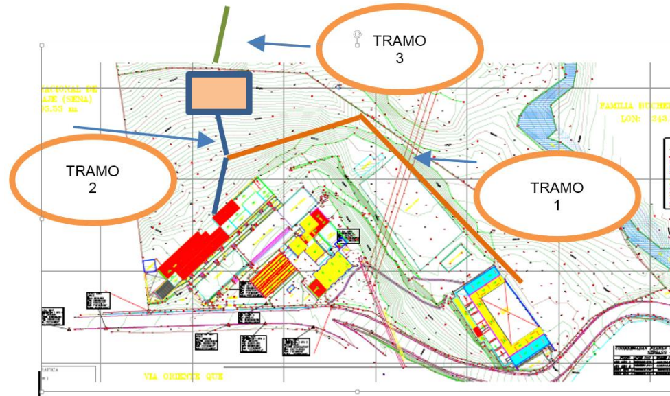
Figura 1. Esquema del sistema de recolección y transporte de aguas residuales hasta la PTAR
