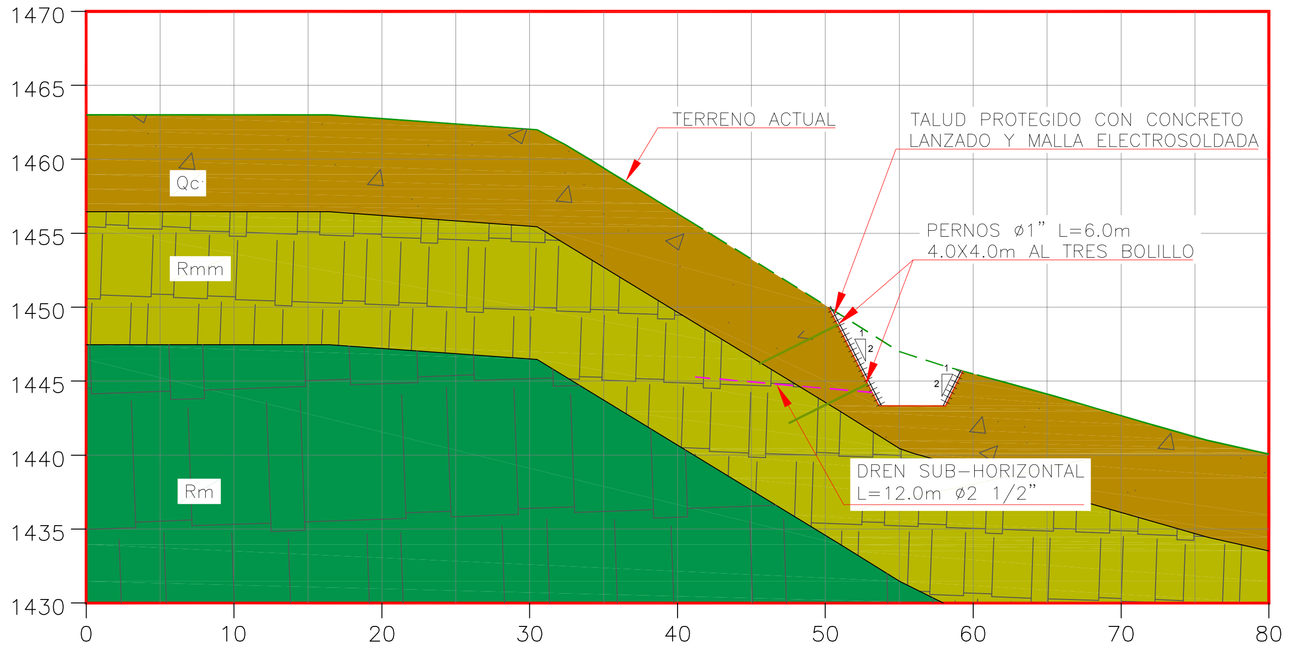
SECCIÓN K 0+257.00 ESC. 1:250
