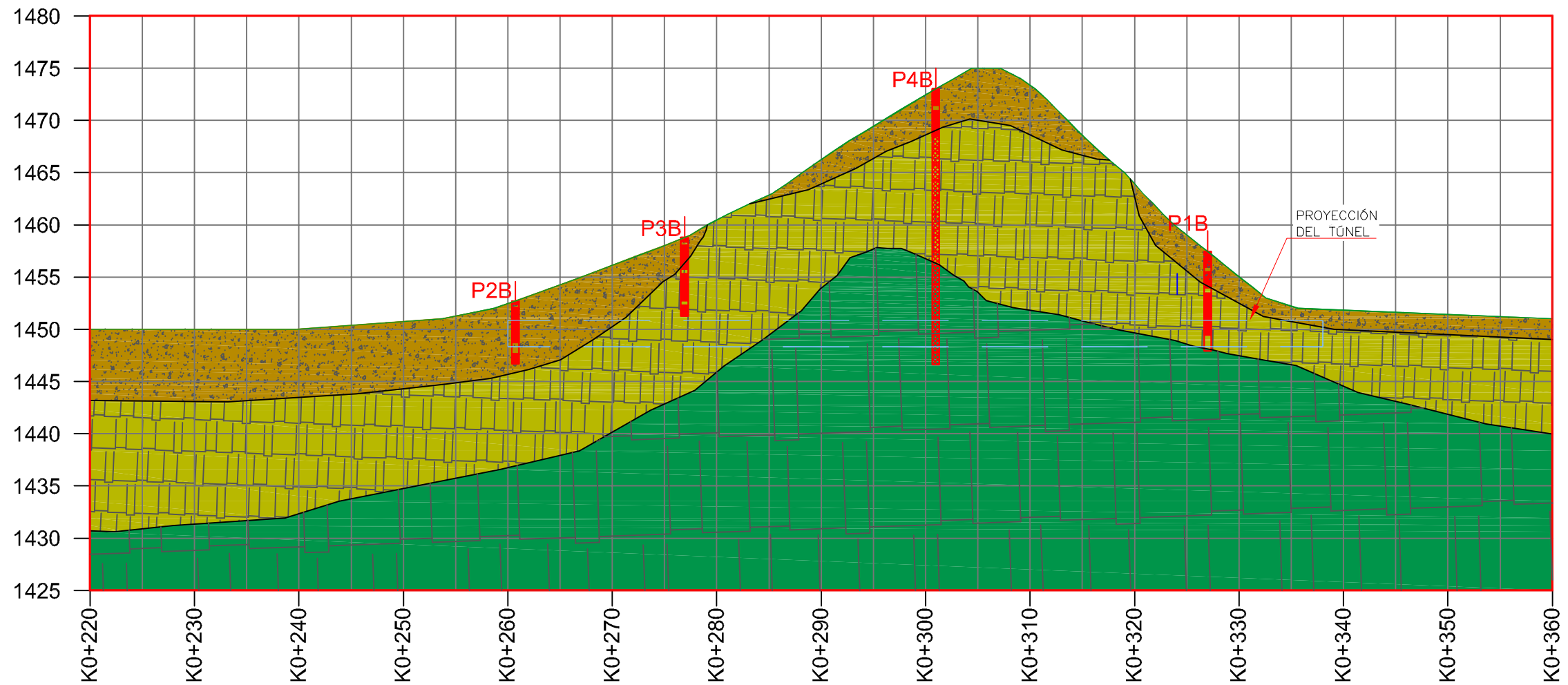
PERFIL A - A' ESC 1:500
