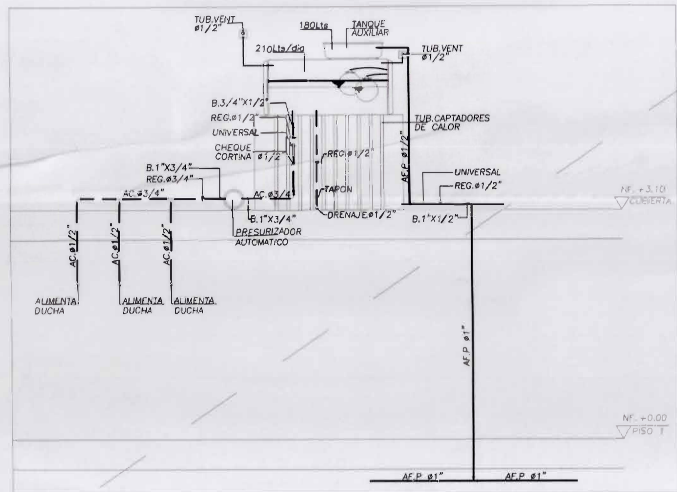
ESQUEMA SISTEMA RADIACION SOLAR Suministro Escala 1:50
