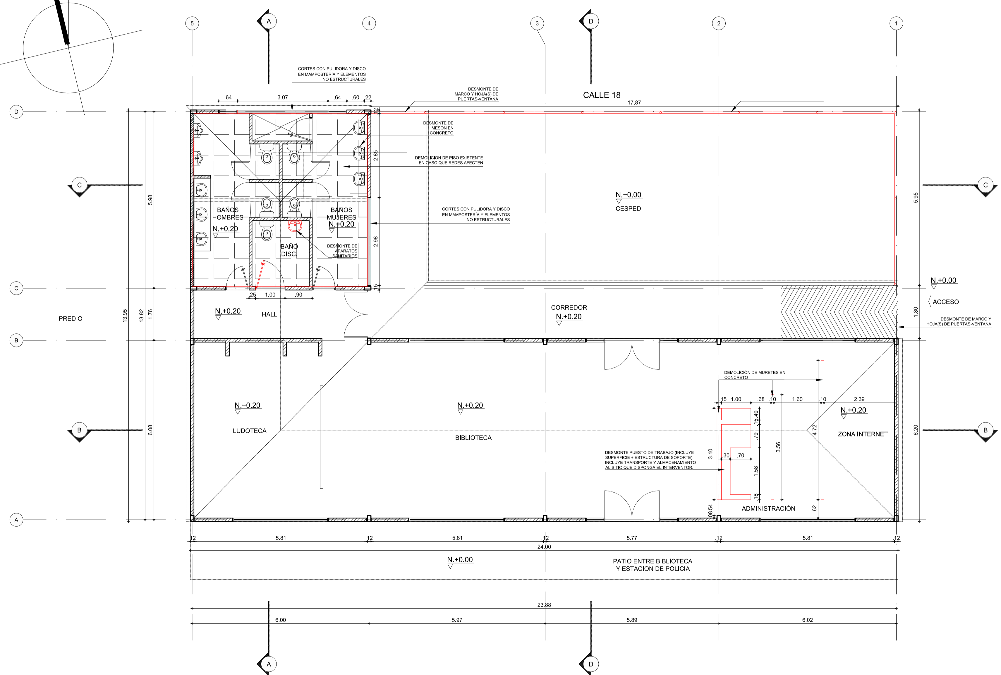
PLANTA DE DEMOLICIONES ESC. 1:75
