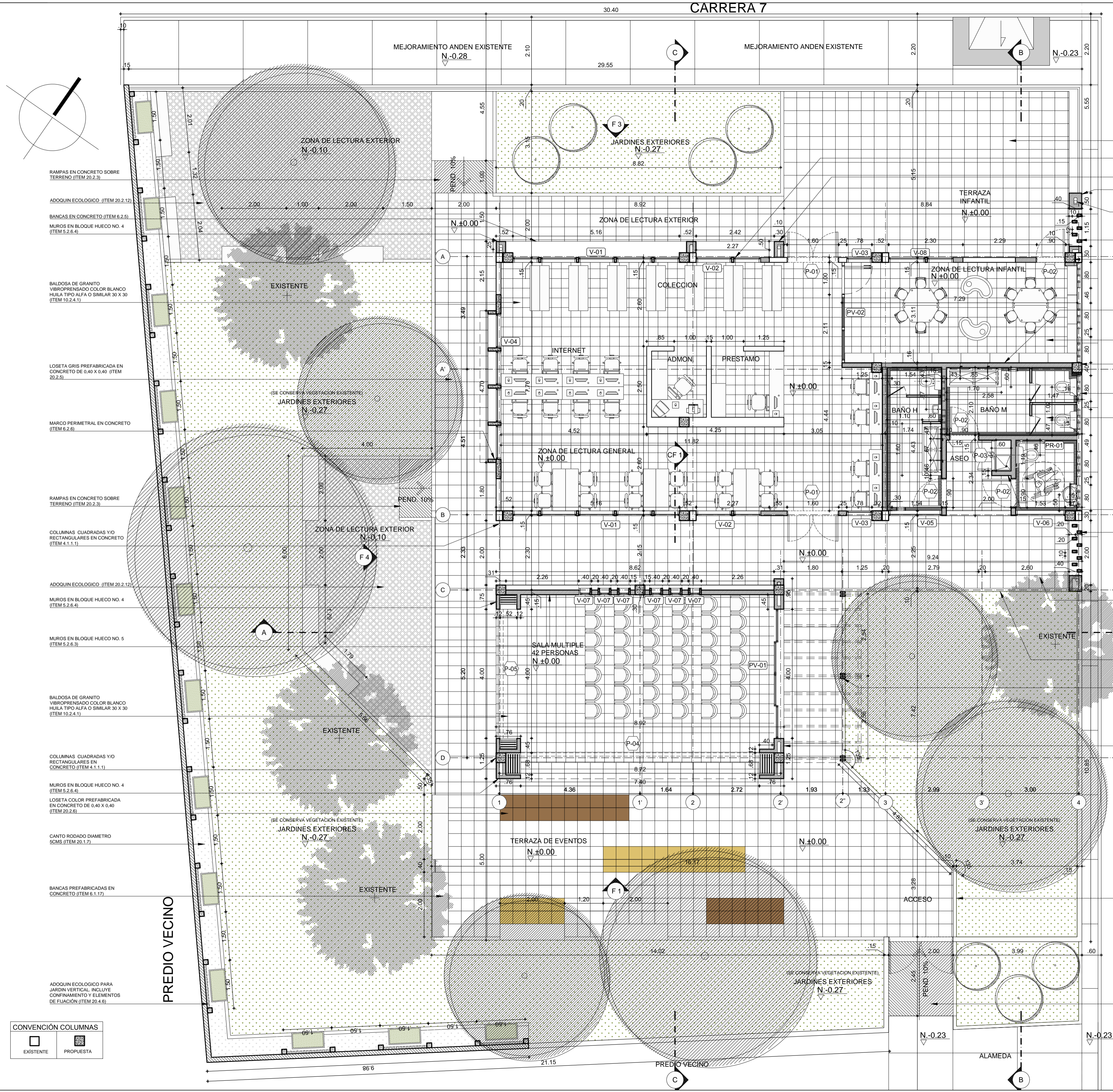
PLANTA PRIMER PISO ESC. 1:75
