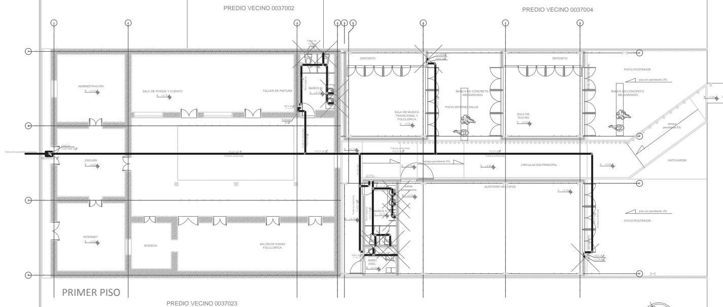
PLANTA PRIMER PISO SUMINISTRO
