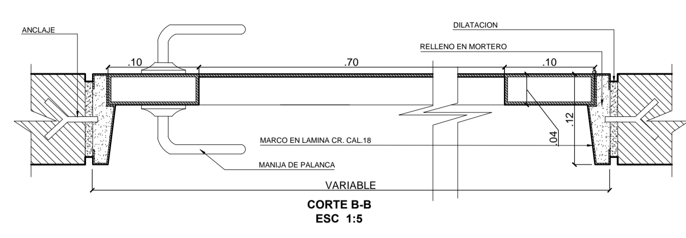
PT-12 DETALLES PUERTA esc. 1:5
