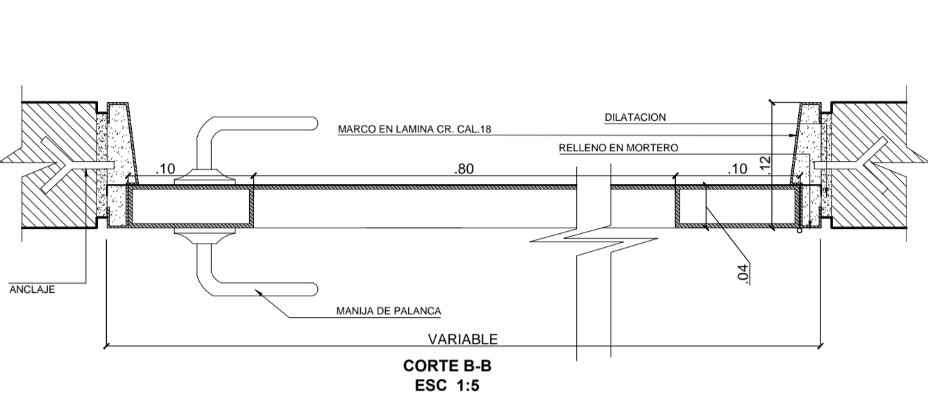
PT-08 DETALLES PUERTA esc. 1:5
