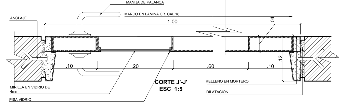
PT-09 DETALLES PUERTA esc. 1:5
