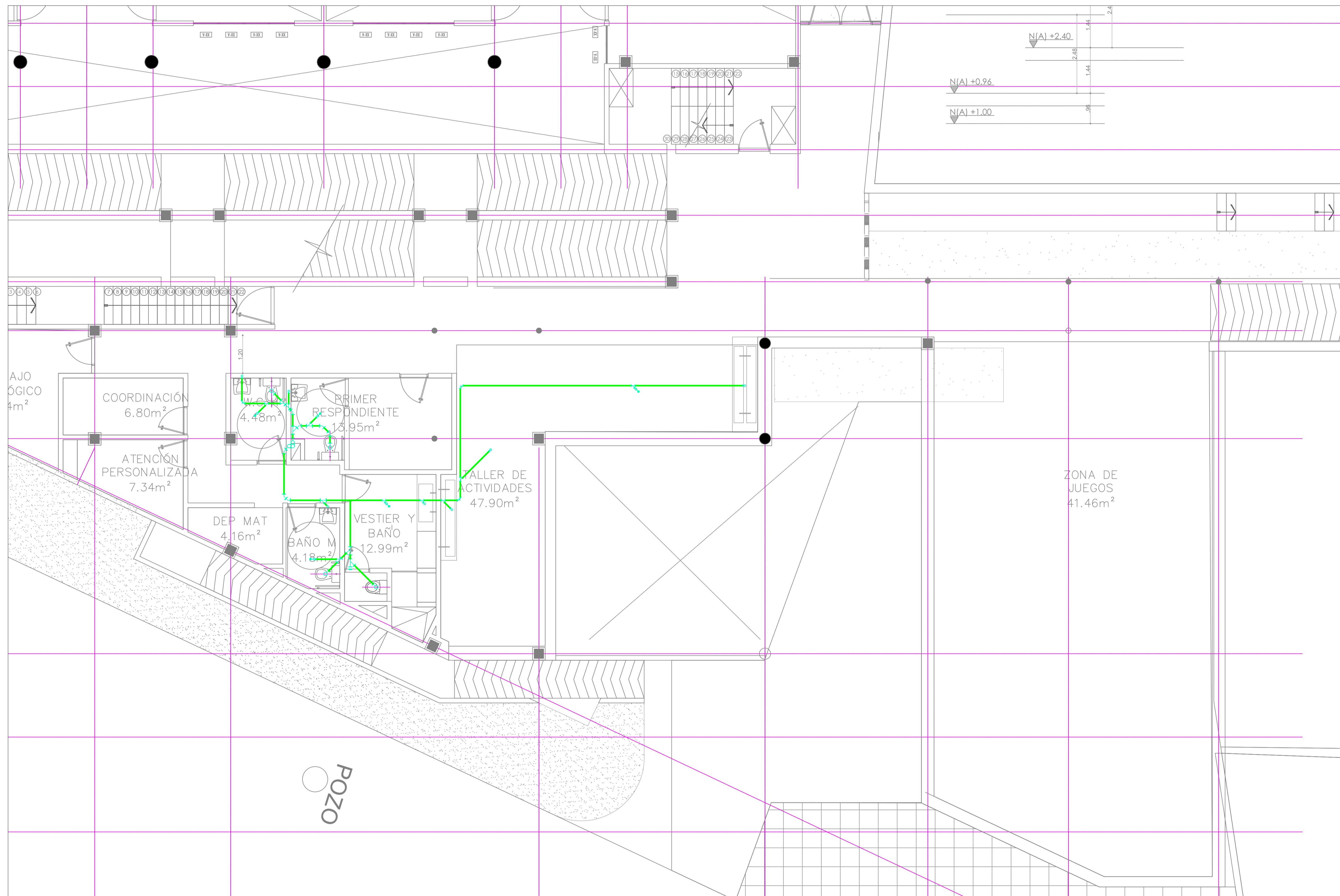
PLANTA GENERAL DESAGUES RE DE DESAGUES ESCALA 1:75
