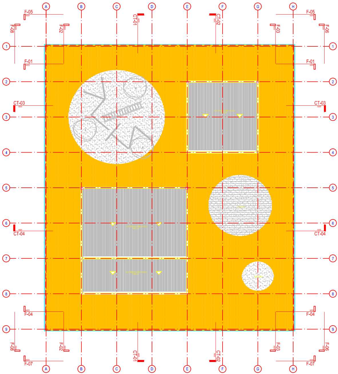
PLANTA CUBIERTAS ESCALA 1:100
