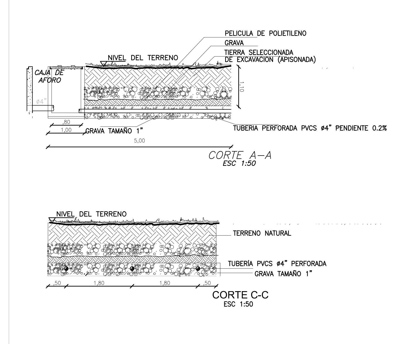
DETALLE CAMPO INFILTRACIÓN ESC_ 1:50
