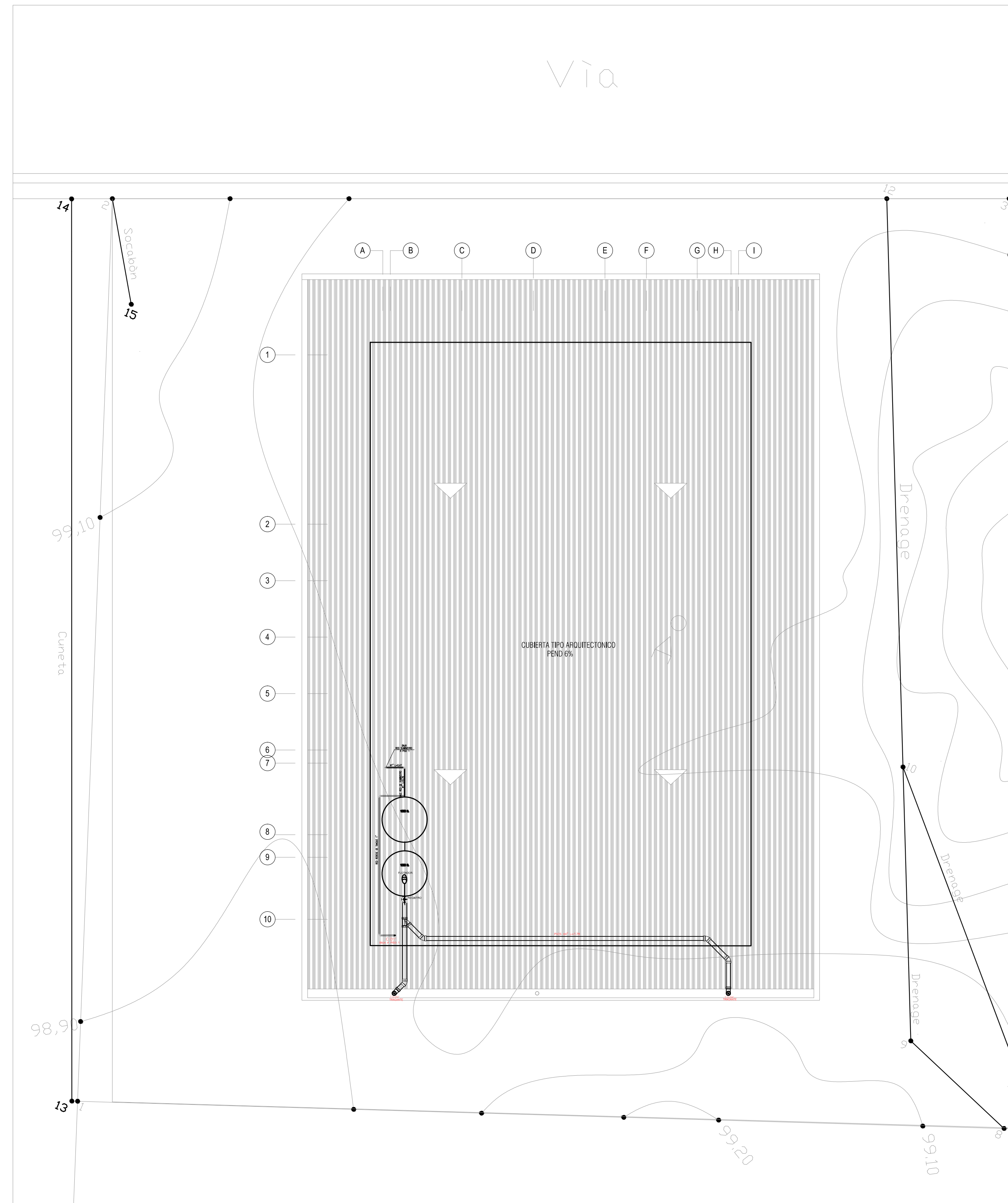
PLANTA DESAGÜES ESC_ 1:75
