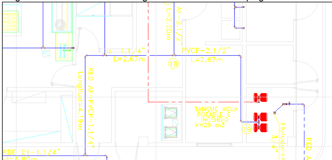
Figura 09. Descarga del equipo de suministro hacia las redes generales
