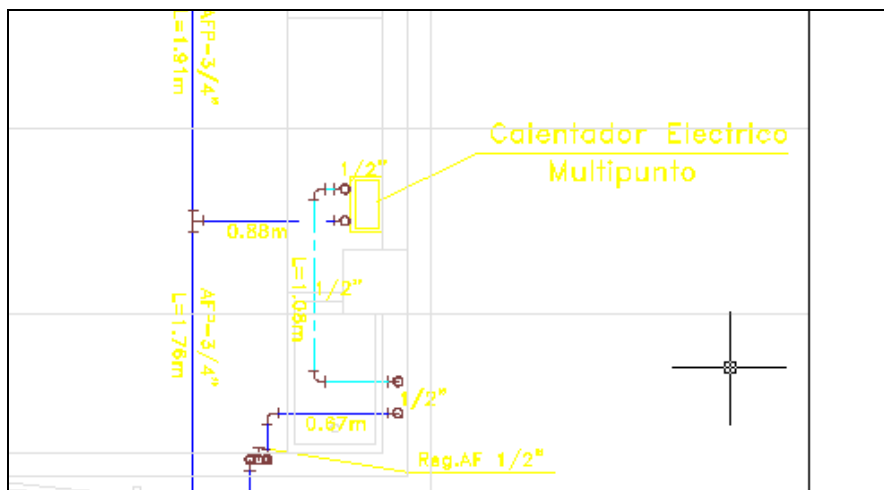
Figura 10.Lavacolas con suministro de Agua Caliente
