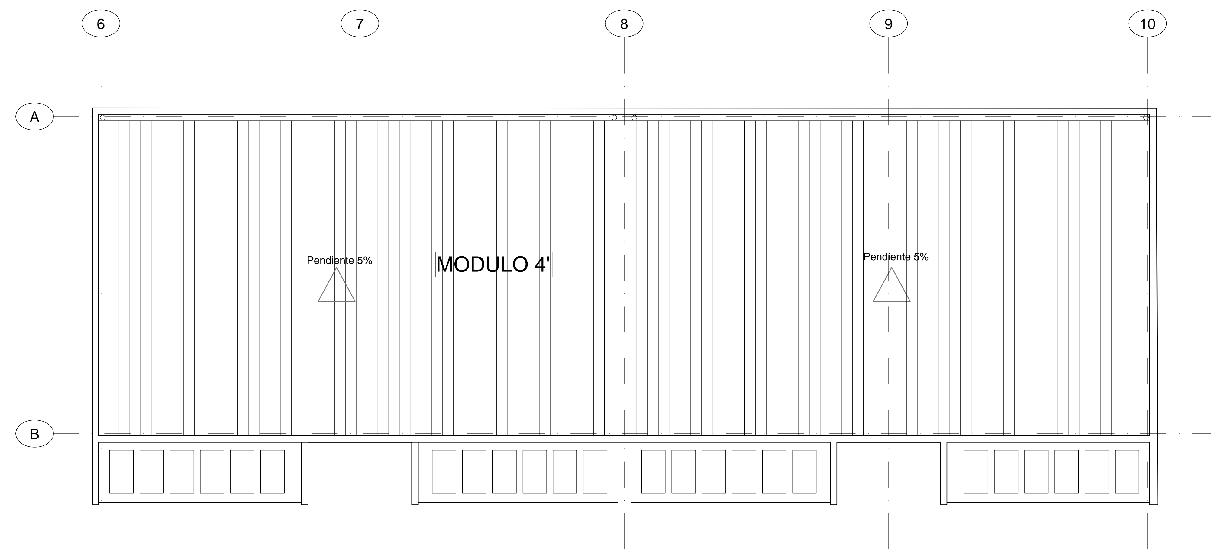
PLANTA DE CUBIERTA ESC. 1:75
