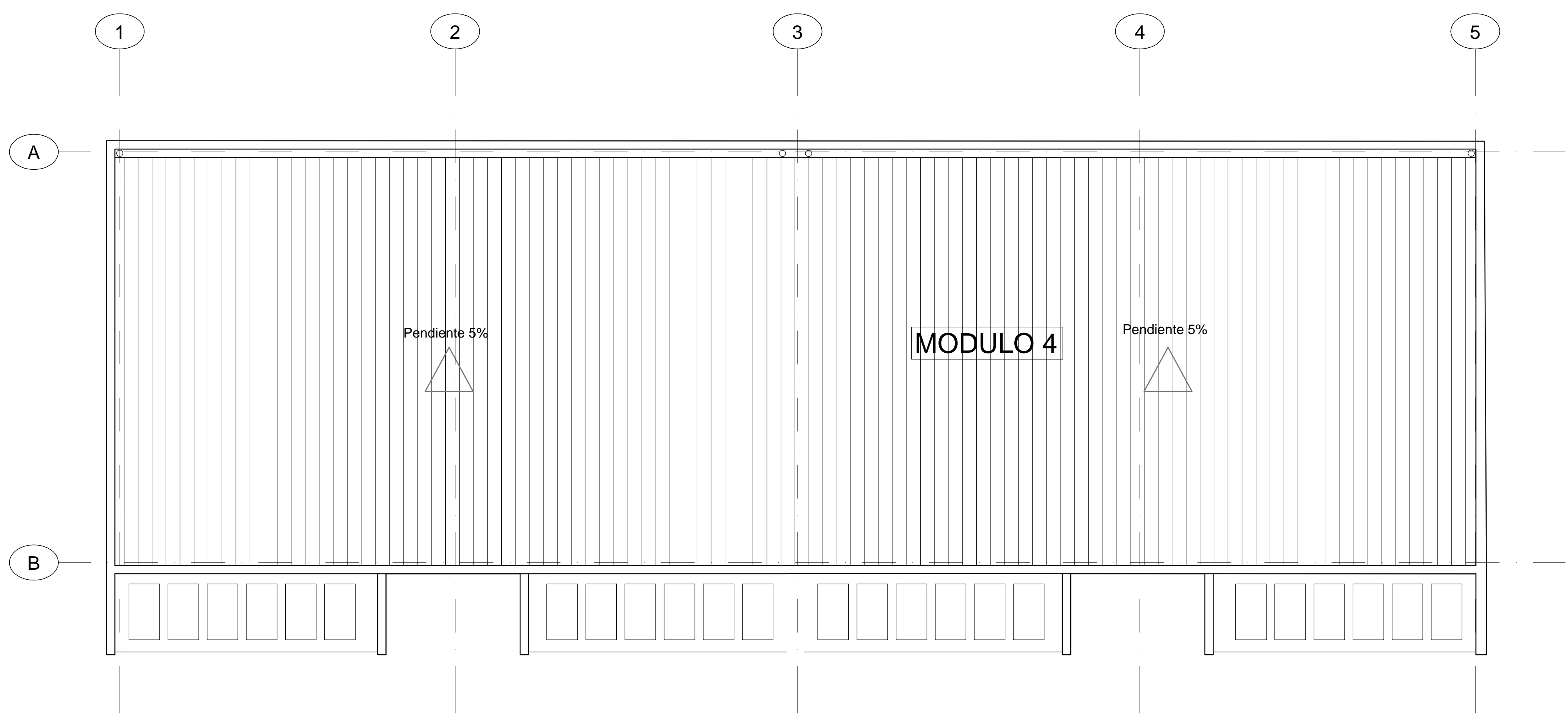
PLANTA DE CUBIERTA ESC. 1:75
