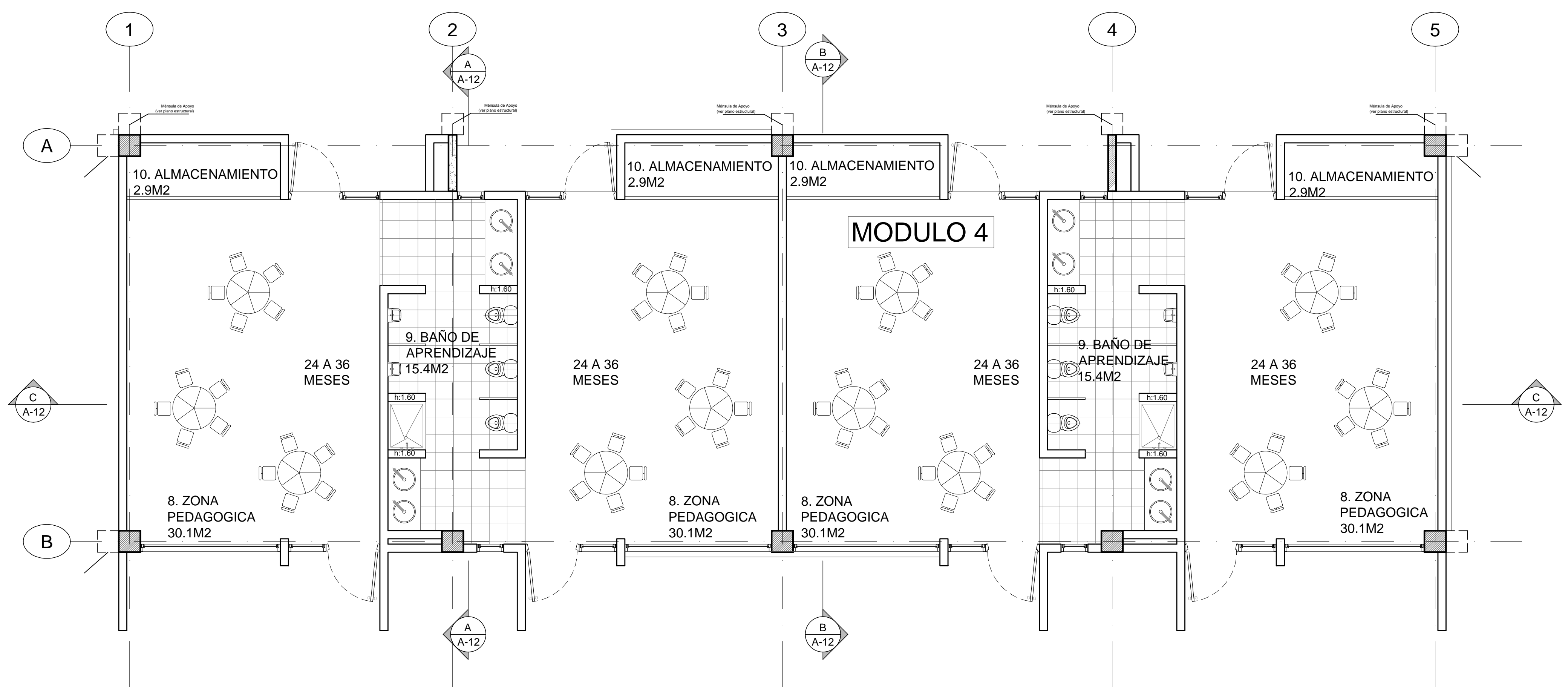
PLANTA ARQUITECTONICA ESC. 1:75
