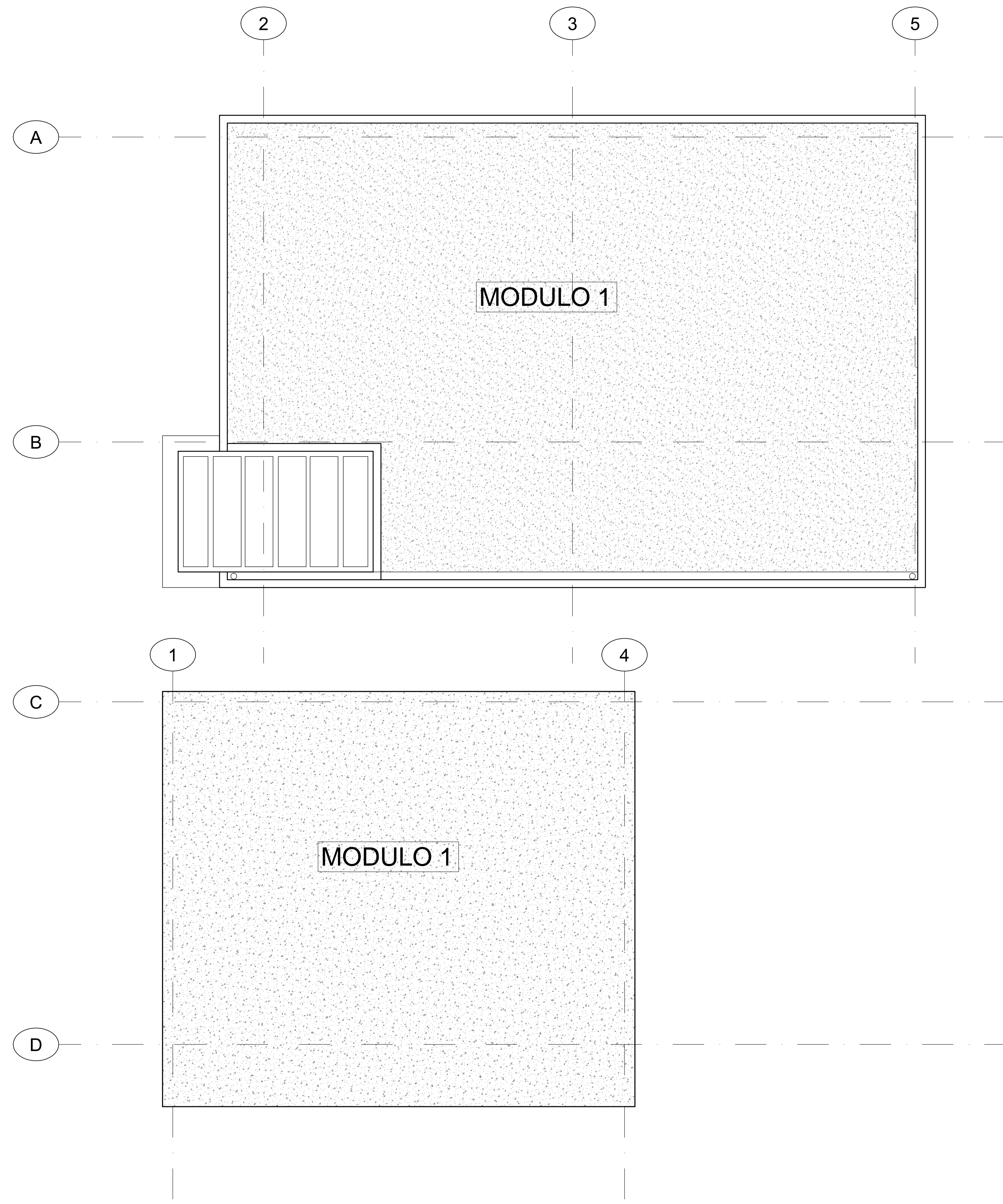
PLANTA DE CUBIERTA ESC.____ 1:75
