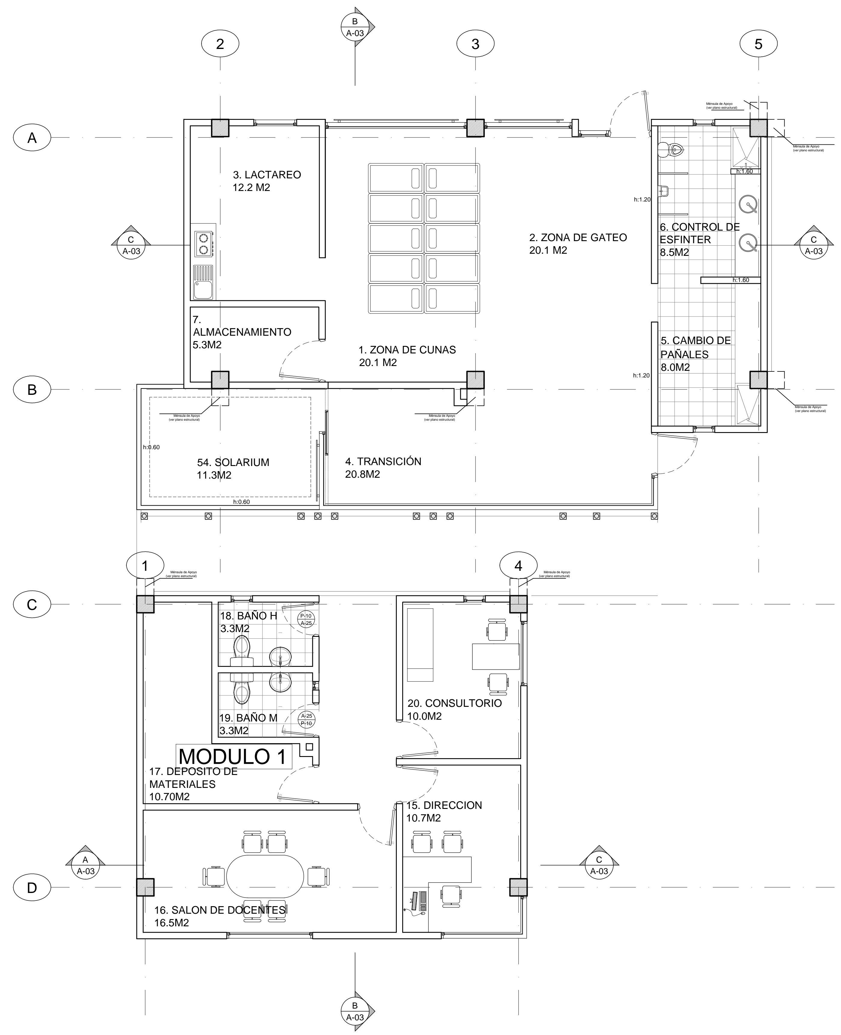
PLANTA ARQUITECTONICA ESC.____ 1:75
