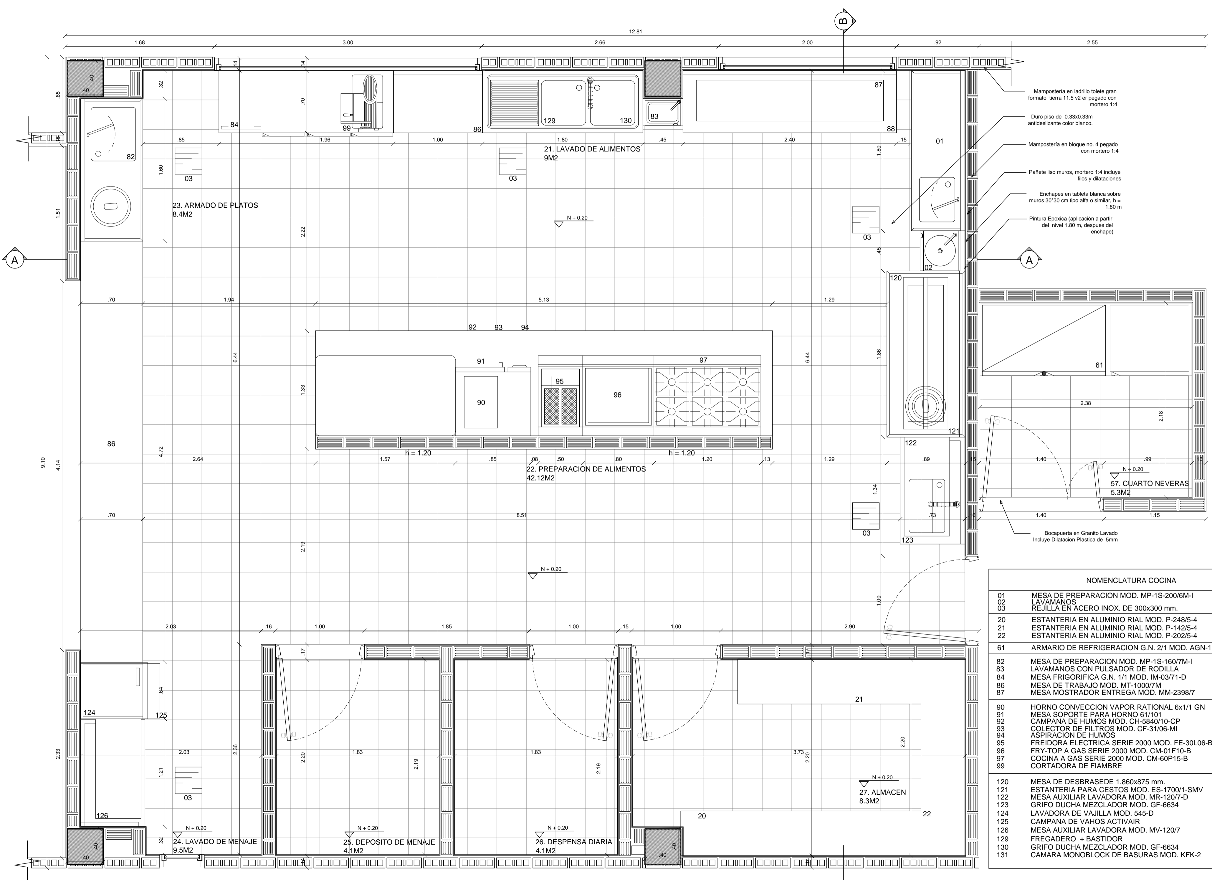
PLANTA COCINA MODULO 3 ESC. 1:25
