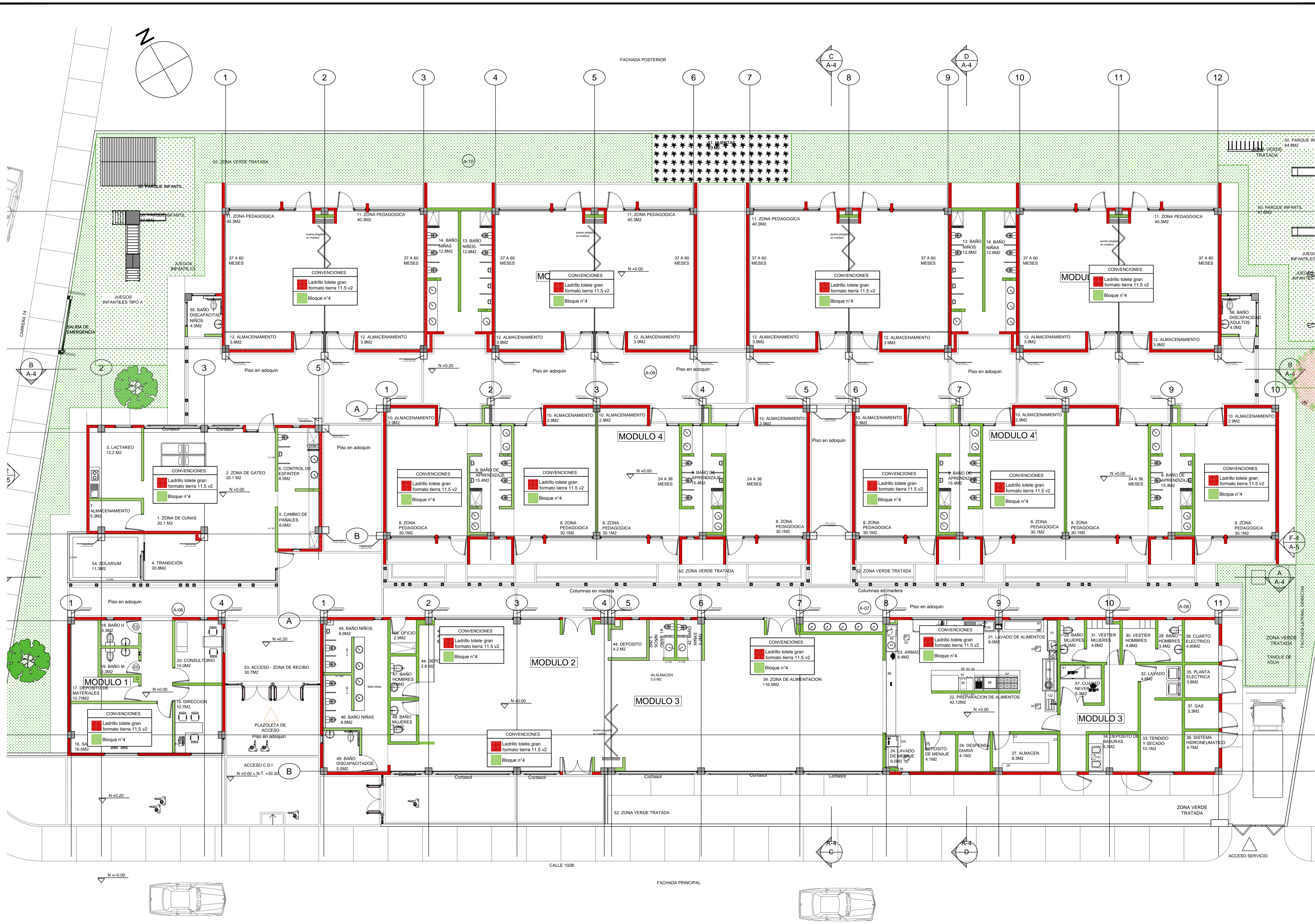
PLANO ESPECIFICACIONES TÉCNICAS MUROS ESC. 1:125
