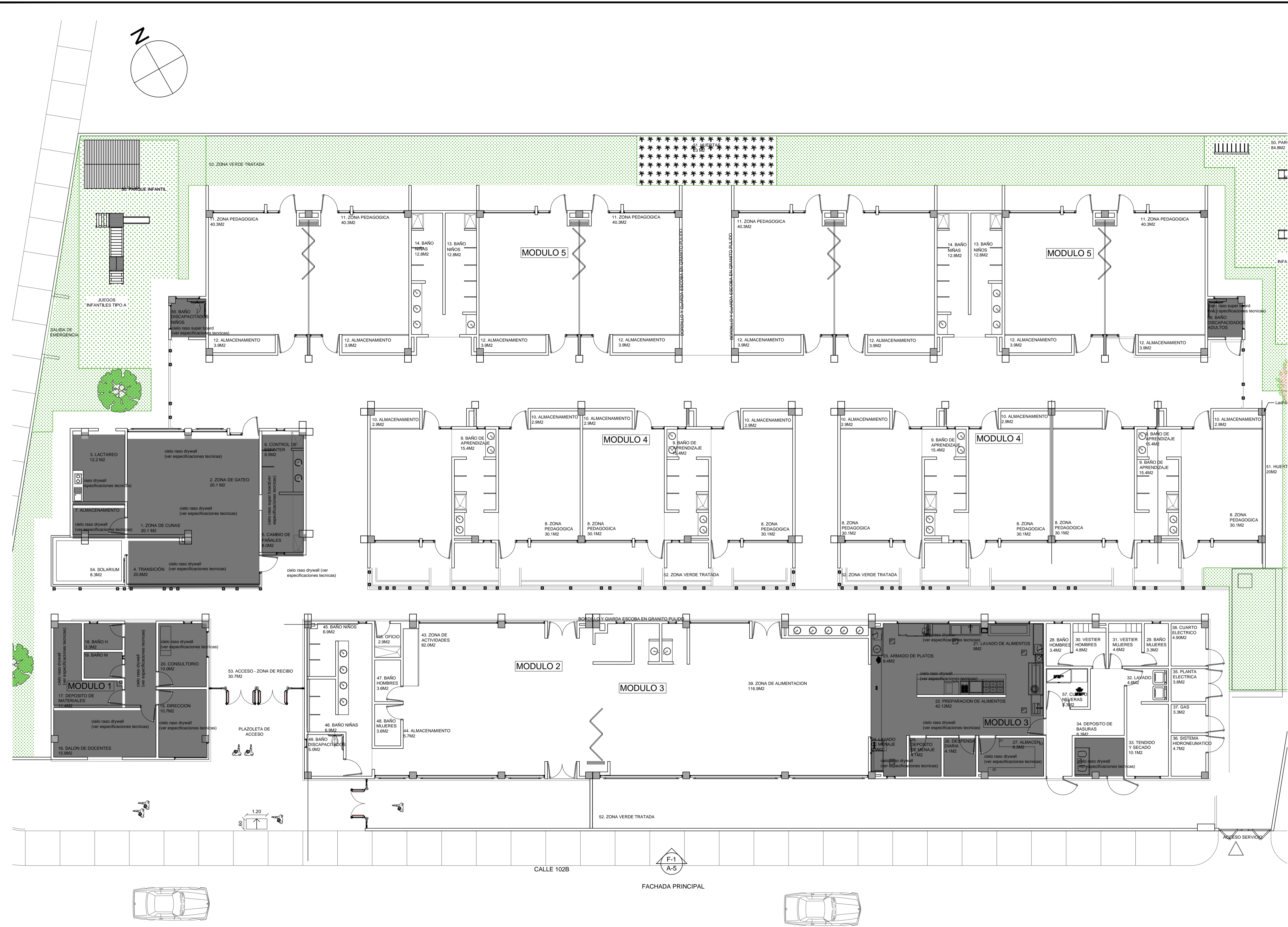
PLANO UBICACIÓN CIELORASO ESC. 1:125
