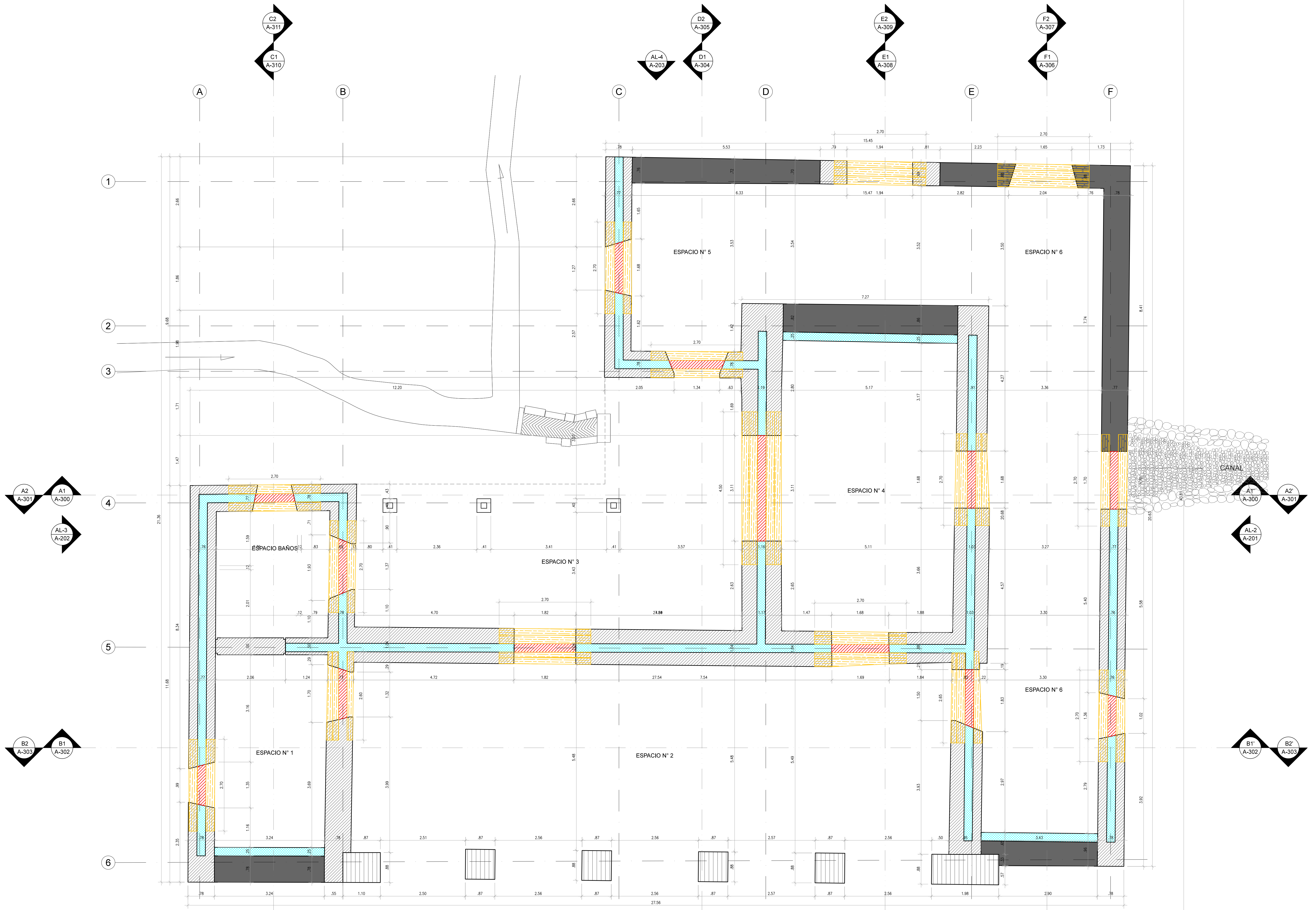
PLANTA DE DINTELES ESC. 1:50
