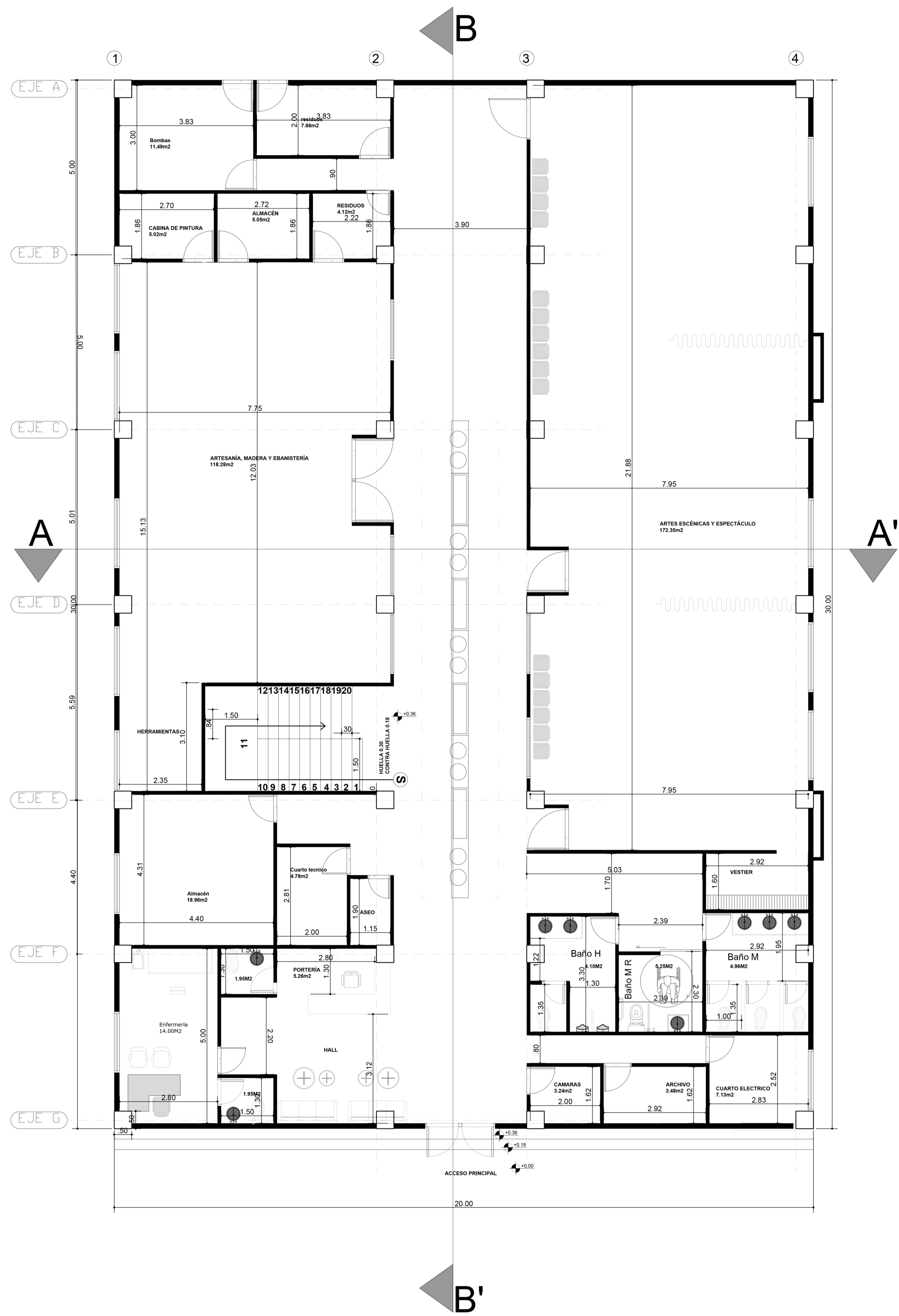
Planta Arquitectónica Primer Piso
