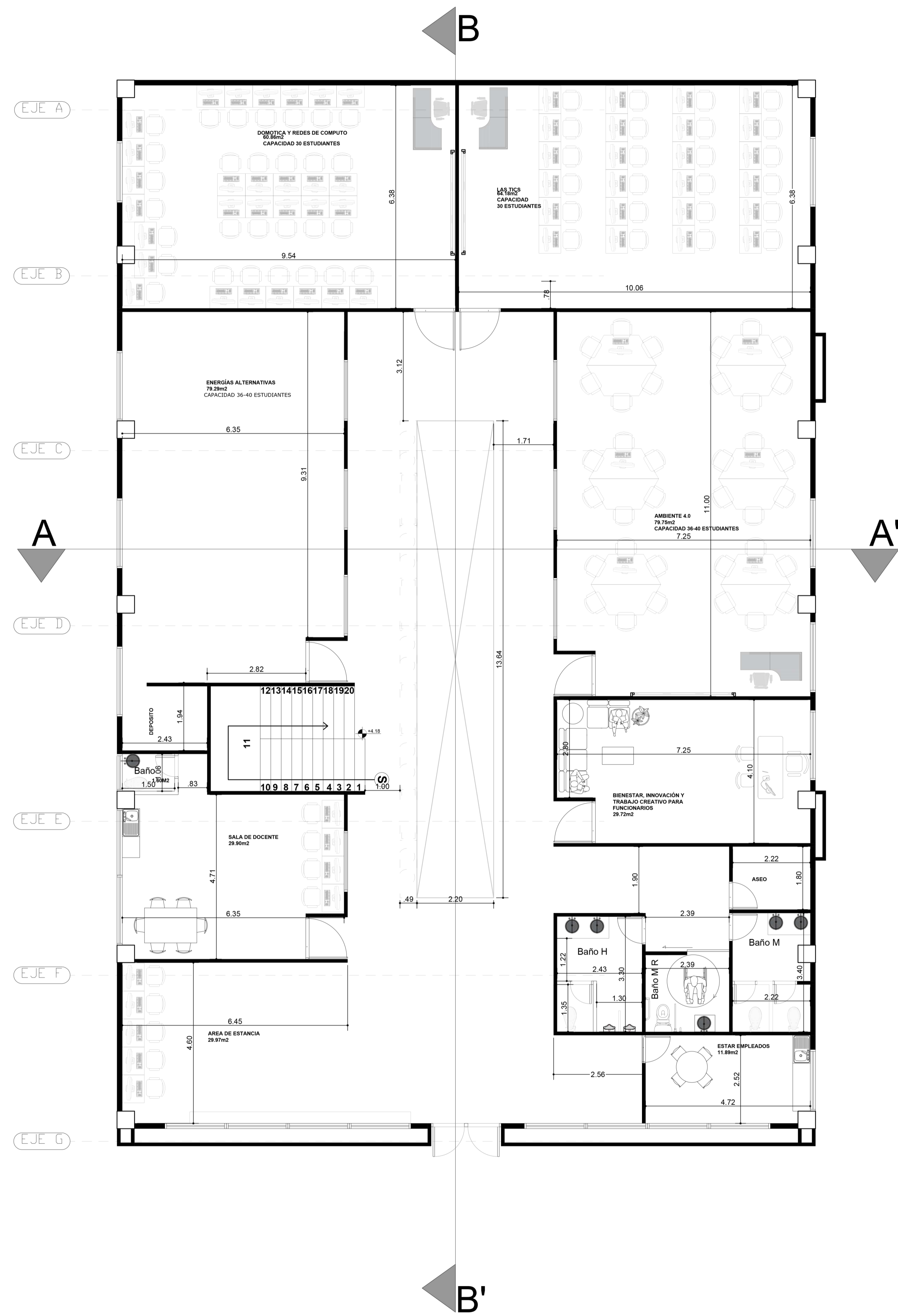
Planta Arquitectónica Segundo Piso
