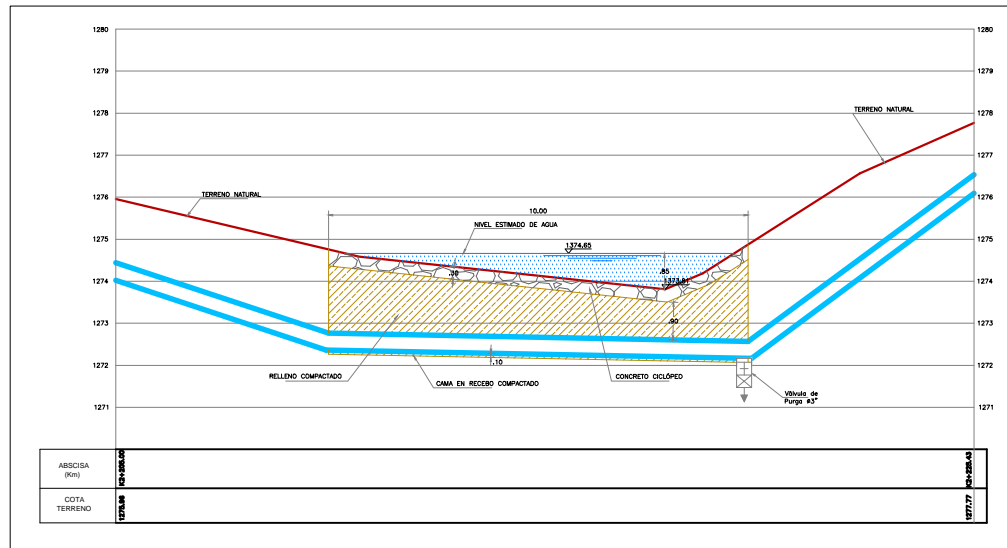
PASO SUBFLUVIAL No. 5 ESC. 1:80
