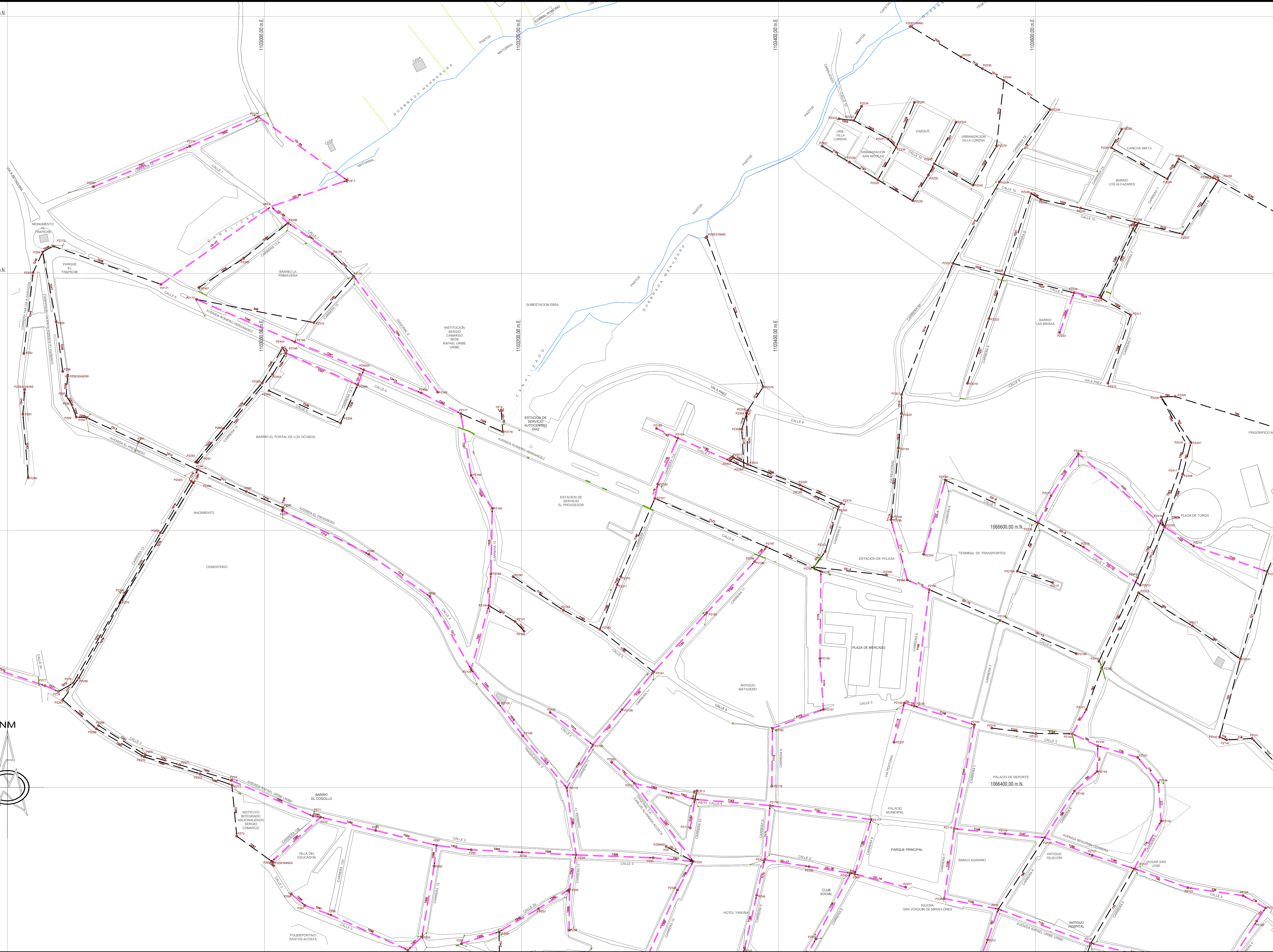
PLANTA PROYECTO ALCANTARILLADO esc 1:1250
