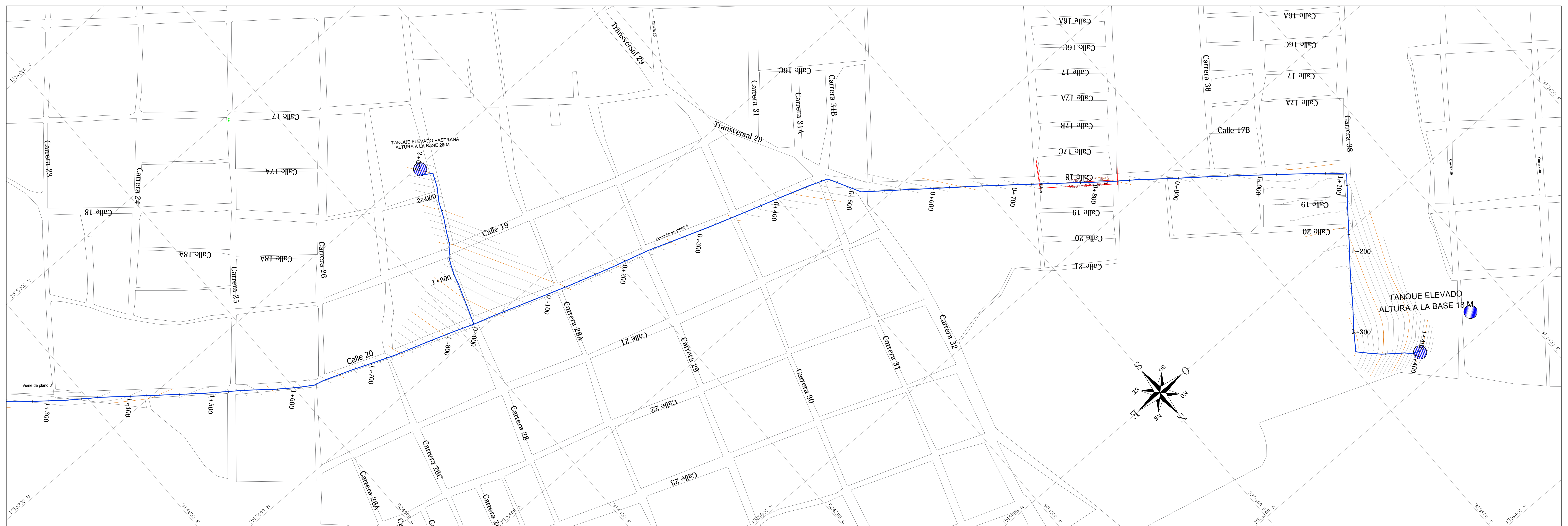
PLANTA PASTRANA-TANQUE 3 ESCALA 1:2000
