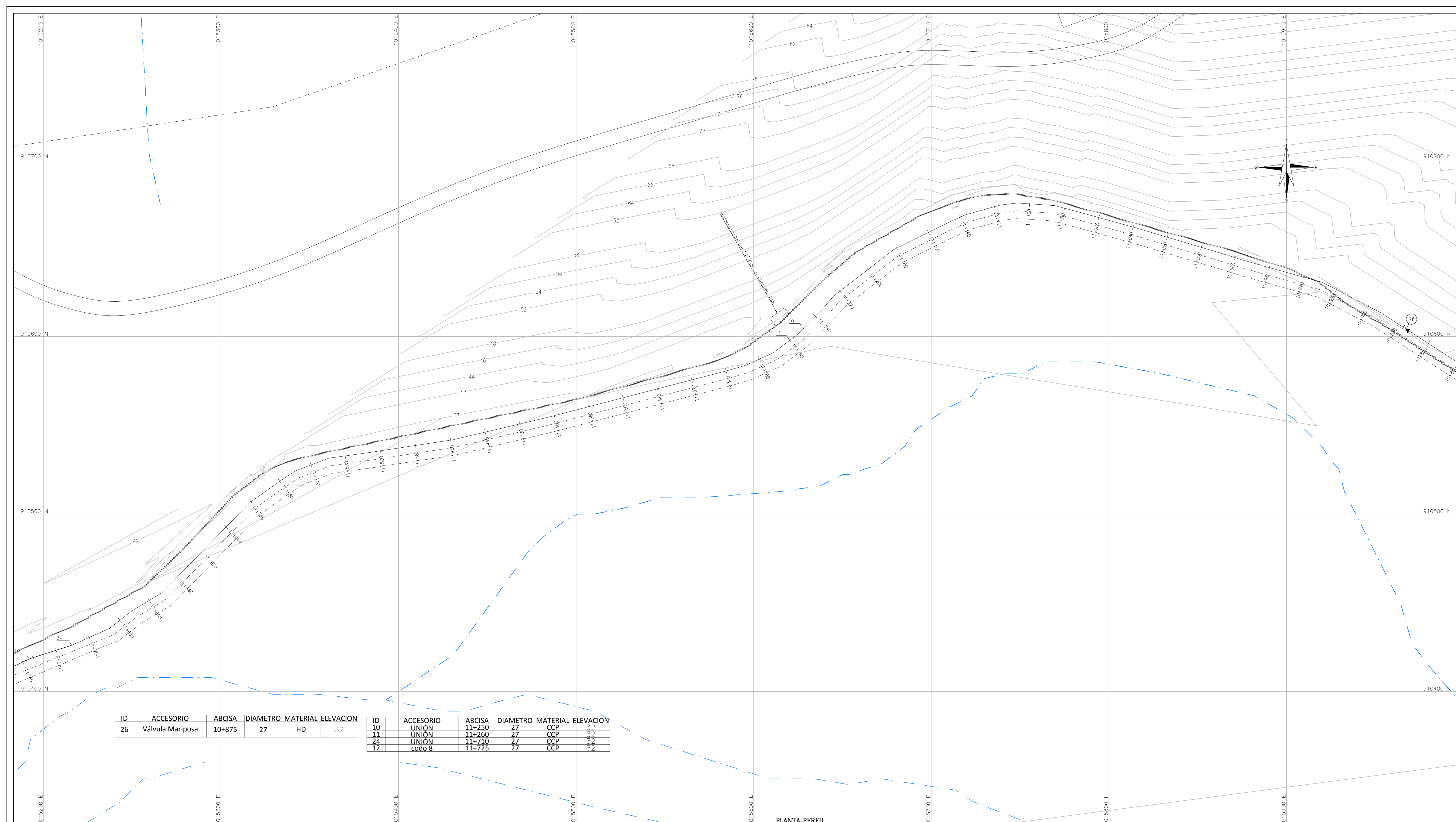
PLANTA-PERFIL ESC 1:1000
