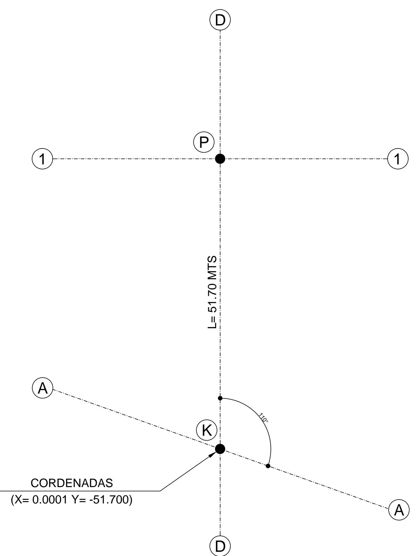
LOCALIZACION EDIFICIO DE OPERACION CON RESPECTO A ESTRUCTURAS HIDRAULICAS ESCALA 1:400
