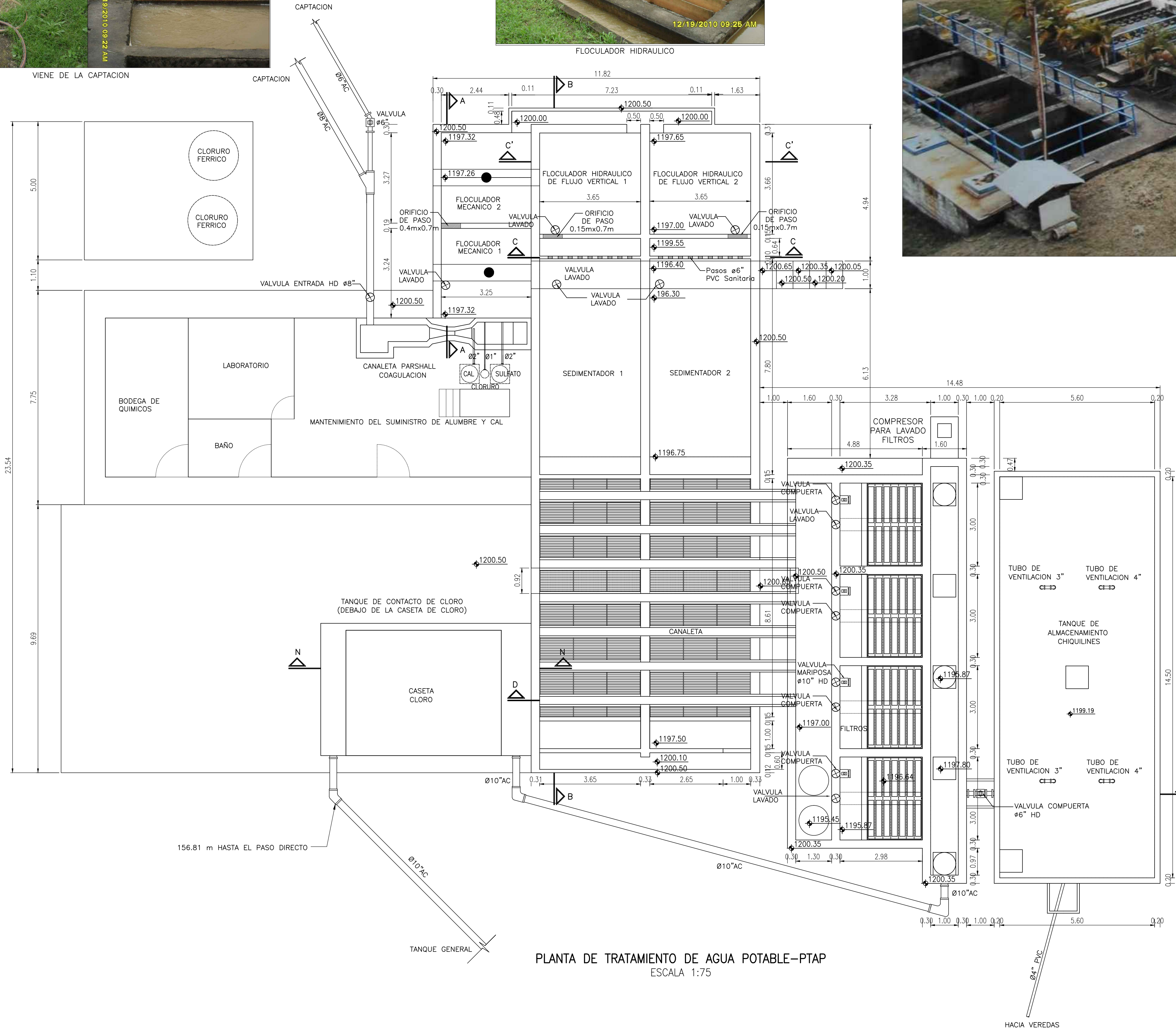
PASARELA FLOCULADOR HIDRAULICO FILTROS
